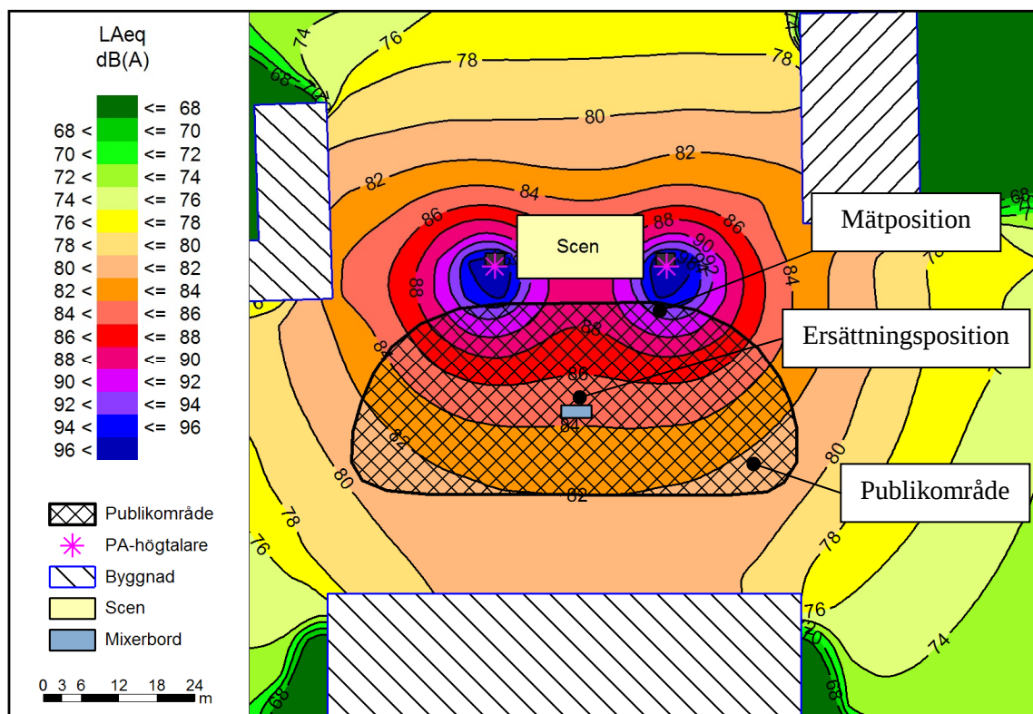
Figur 4 Ljudtrycksnivåer under första timmen vid en utomhuskonsert utritade som ljudnivåkonturer. Val av mätpunkt enligt avsnitt 5.1.1 samt val av ersättningsposition enligt avsnitt 6.1.3
