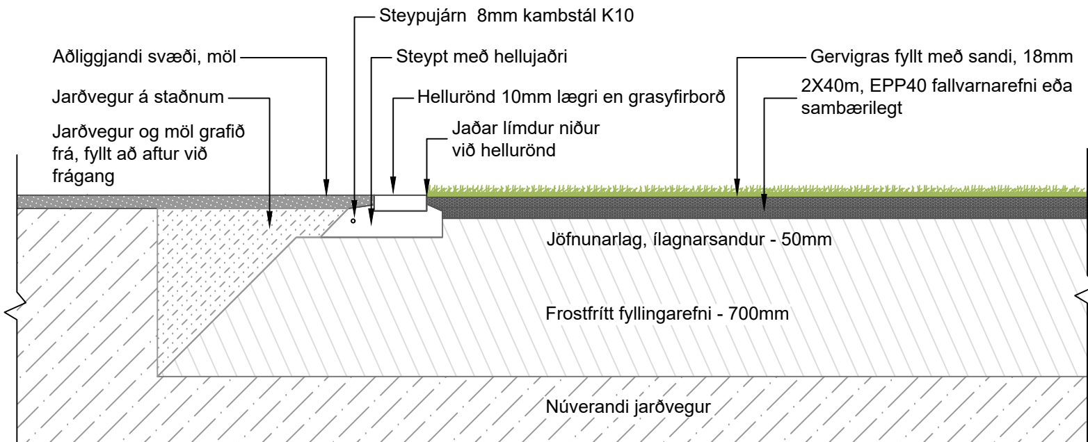
Kennisnið - Fallvörn, gúmmígrasmottur, fallvörn ræðst af fjölda laga. 1:20
