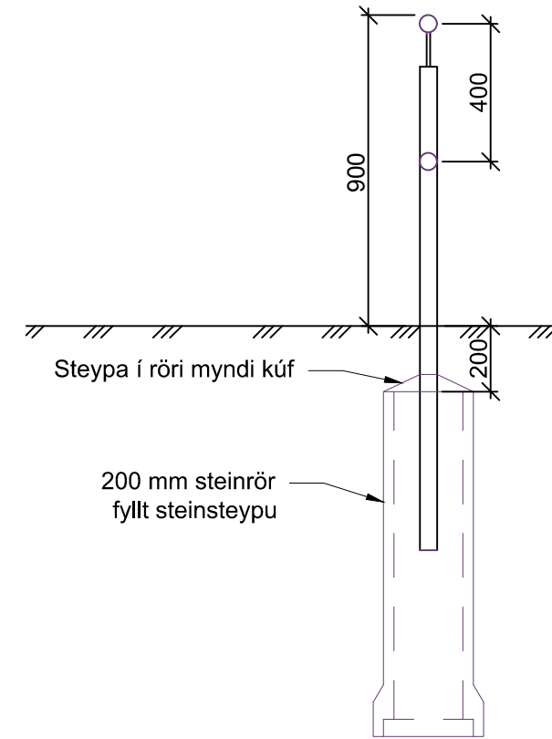
Handrið við útsýnispall - festing handriðsstólpa í jörðu 1:20
