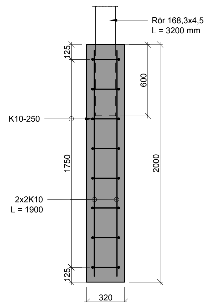
Undirstaða timbur hljóðveggs - deili 1:20
