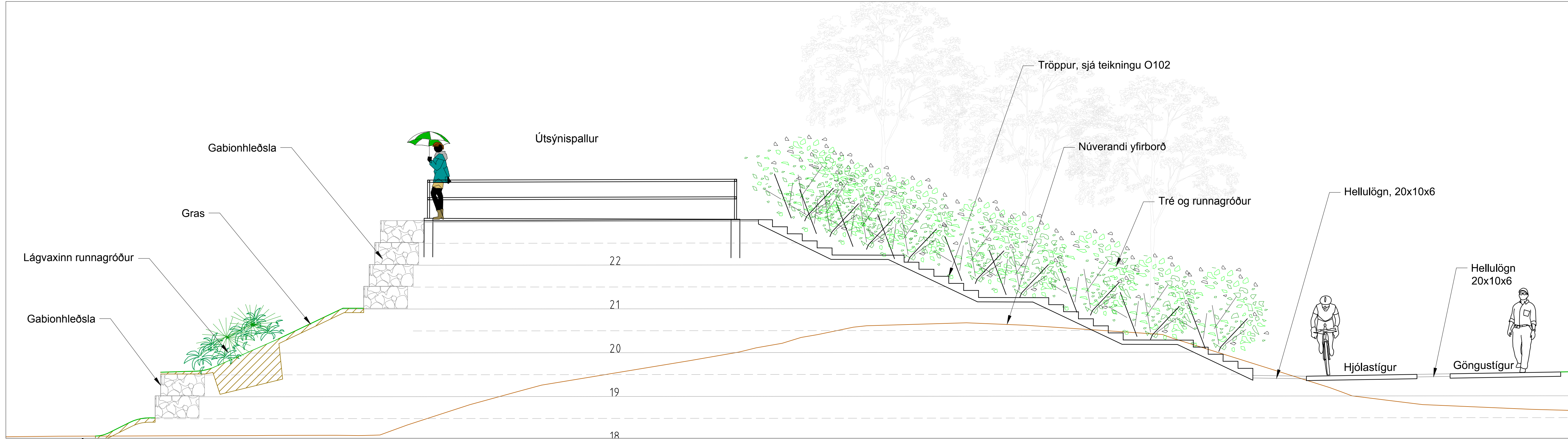
Snið C-C' - Útsýnispallur. 1:50
