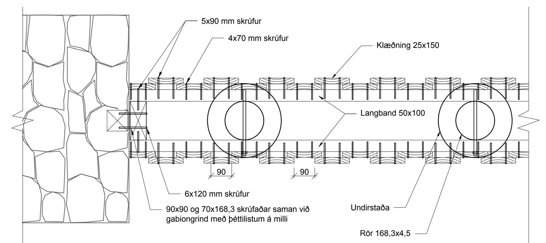
Tenging gabion hljóðveggs og timbur hljóðveggs - deili 1:10
