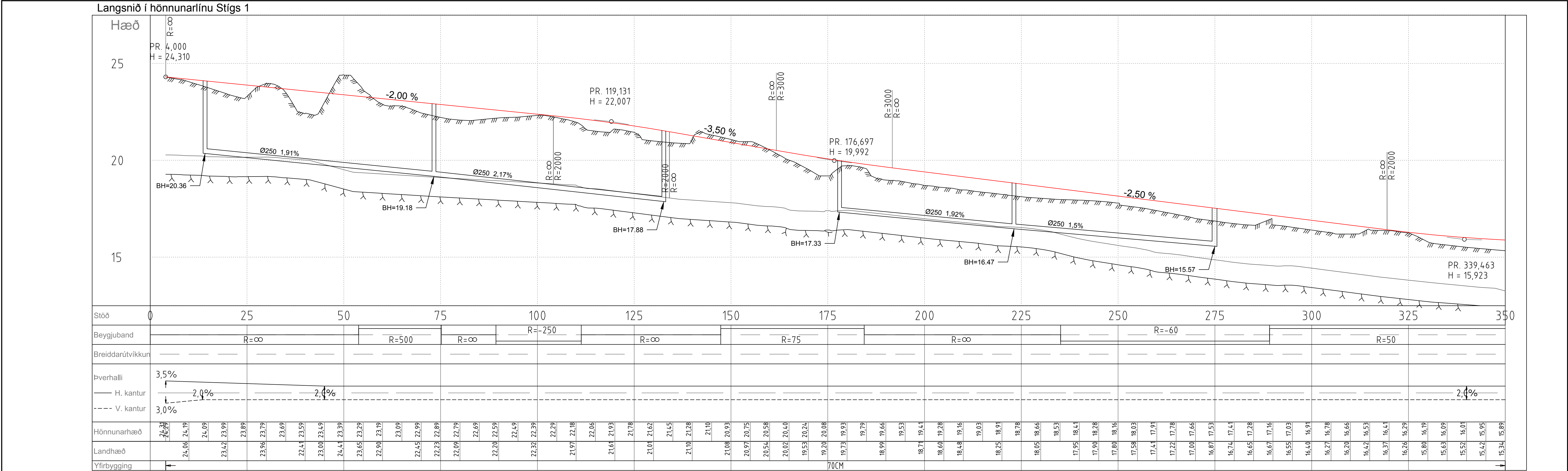
Langsnið 1:500/1:100
