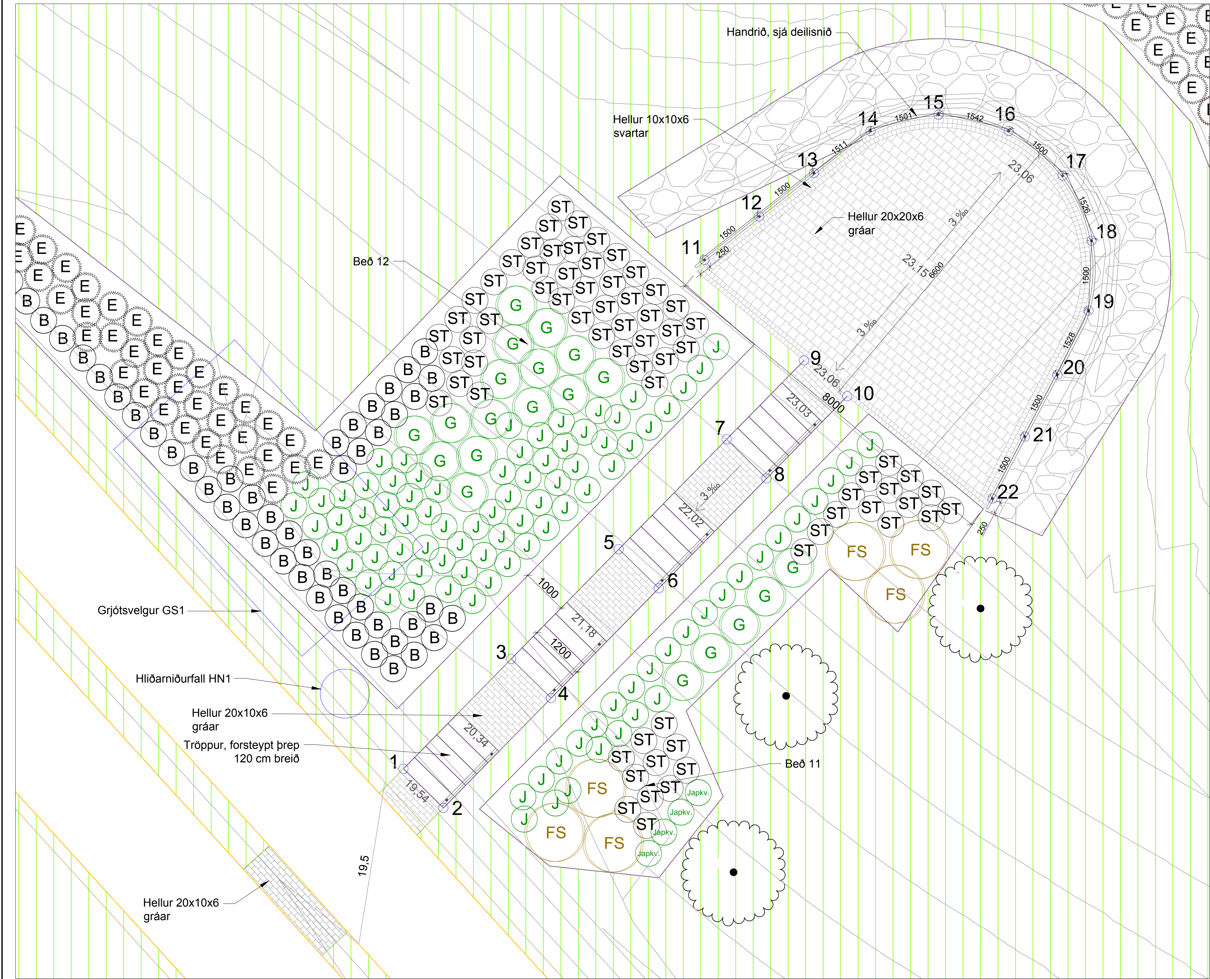
Mynd 1. Útsýnispallur 1:50
