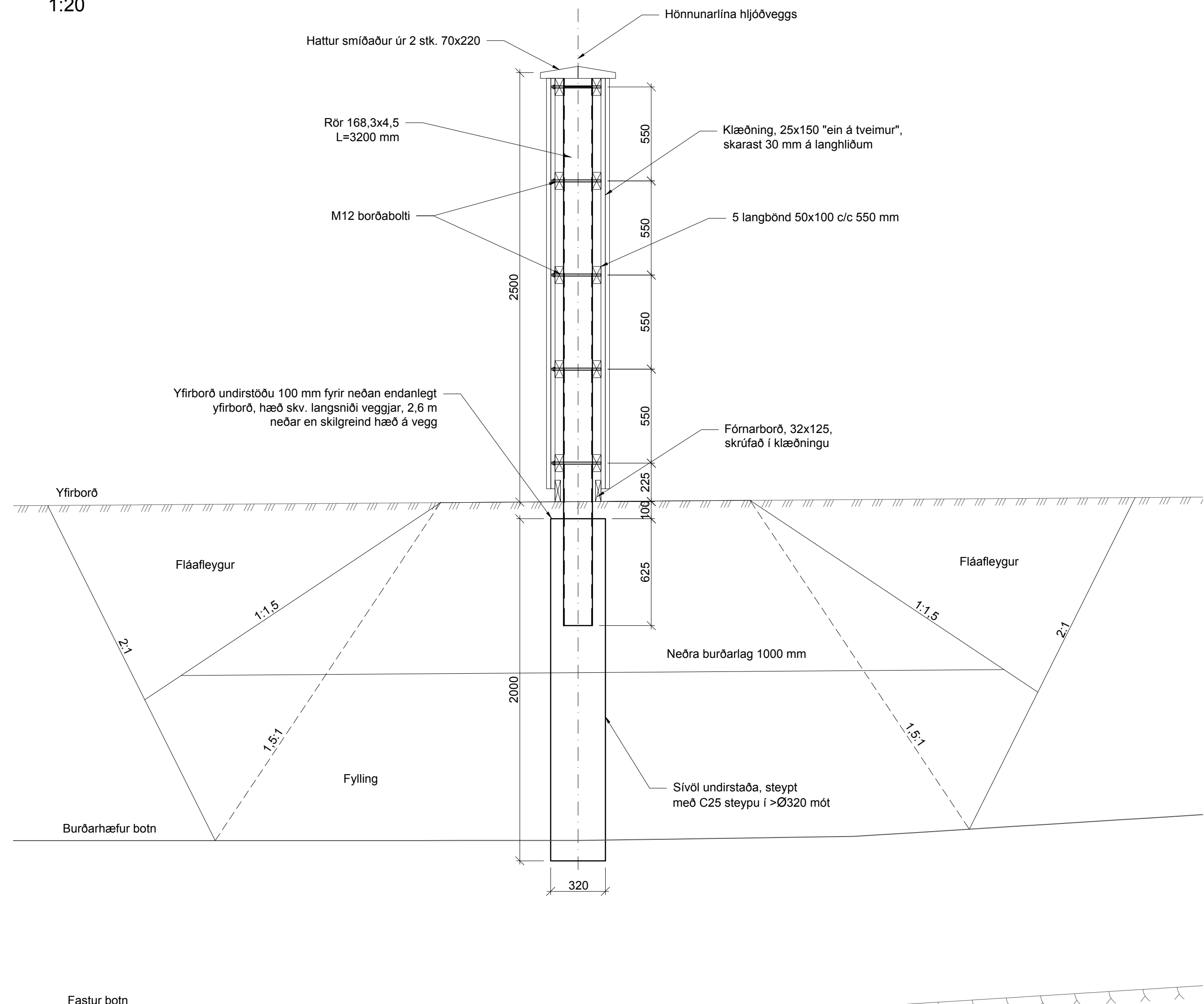
Timbur hljóðveggur - snið 1:20
