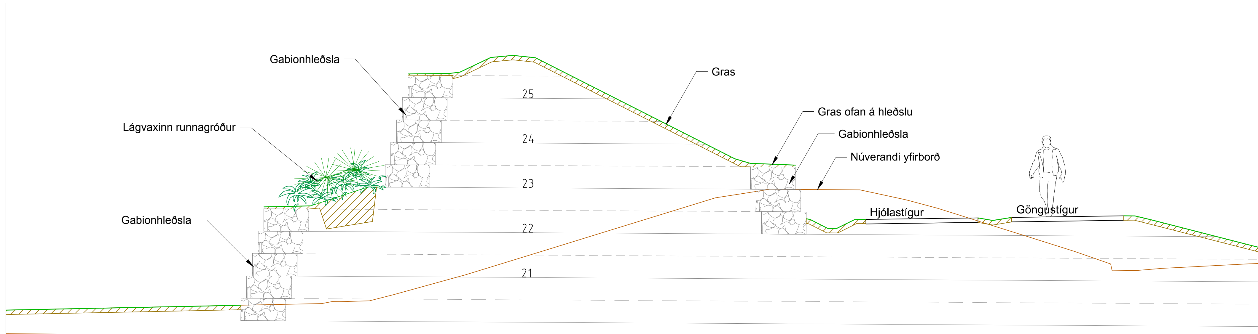
Snið B - B' - Hljóðmön með gabionhleðslu. Gróður á syllu. 1:50
