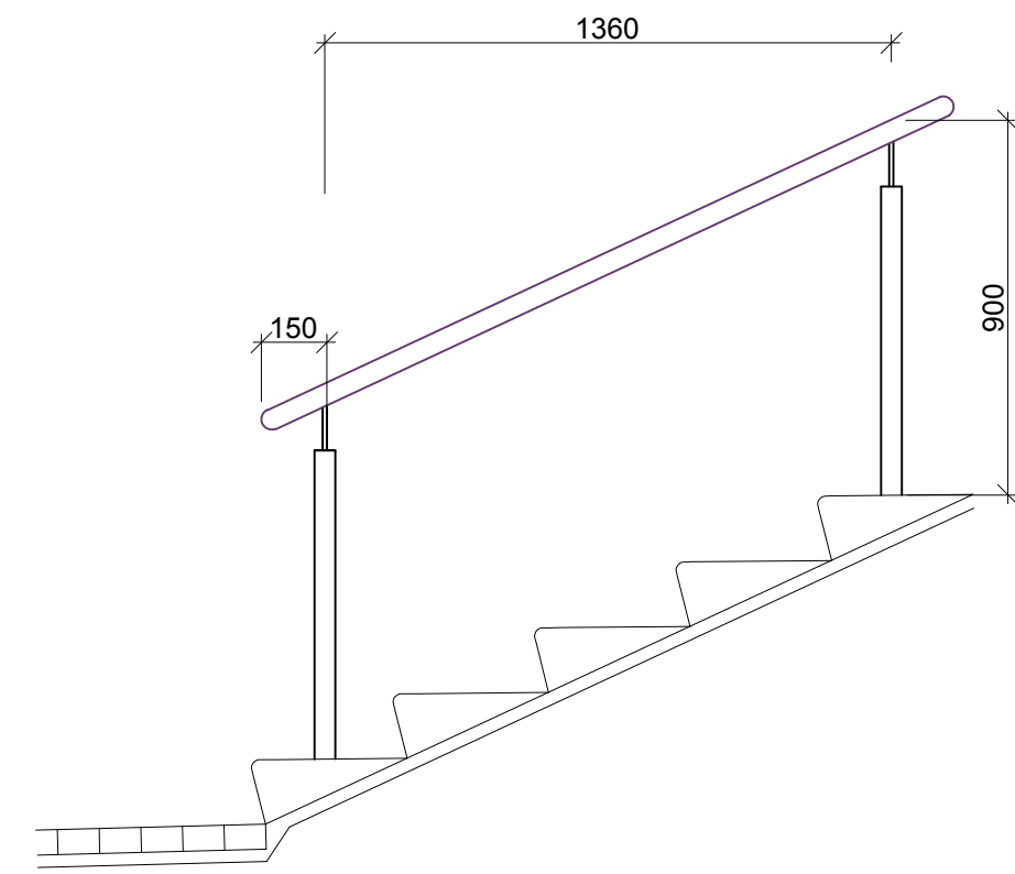
Festing fyrir handriðsstólpa í tröppu 1:10
