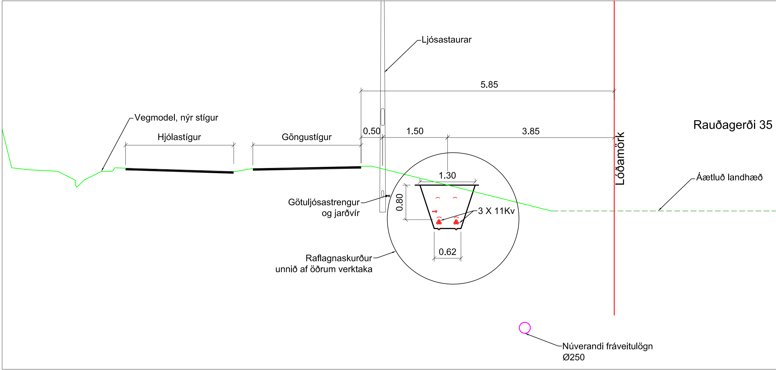
A Snið 1:50
