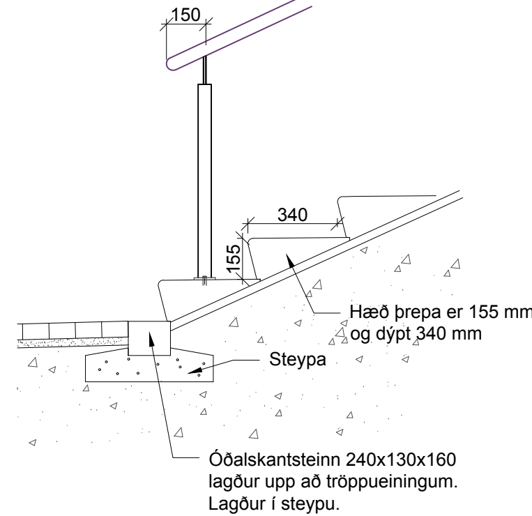
Þrep á tröppum - snið 1:20
