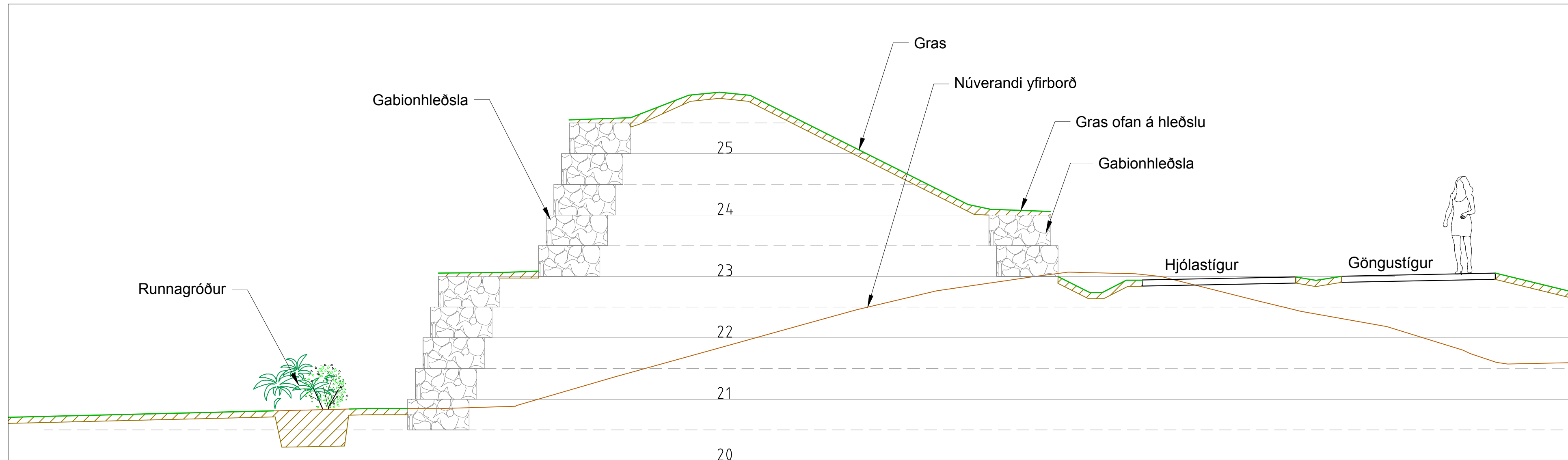
Snið A-A' - Hljóðmön með gabionhleðslu. 1:50
