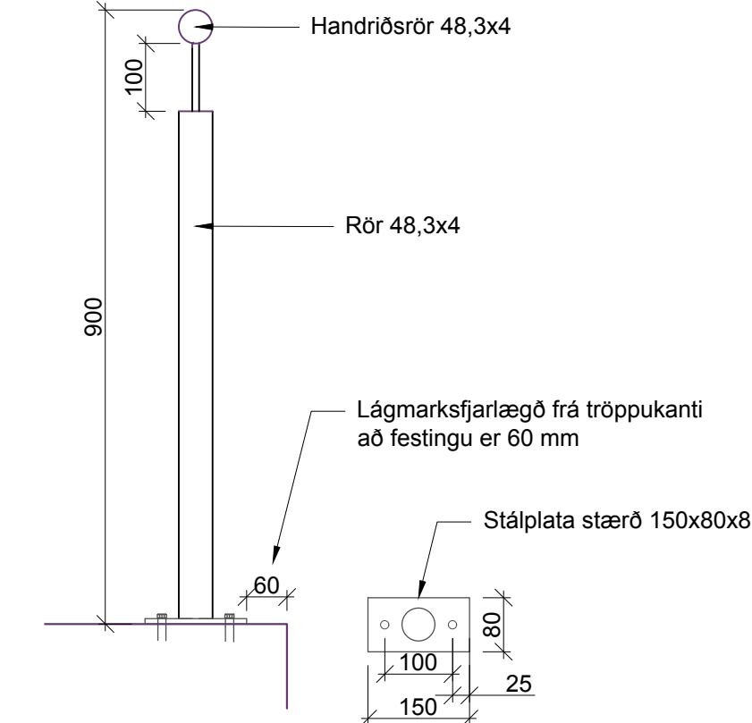
Festing fyrir handriðsstólpa í tröppu 1:10
