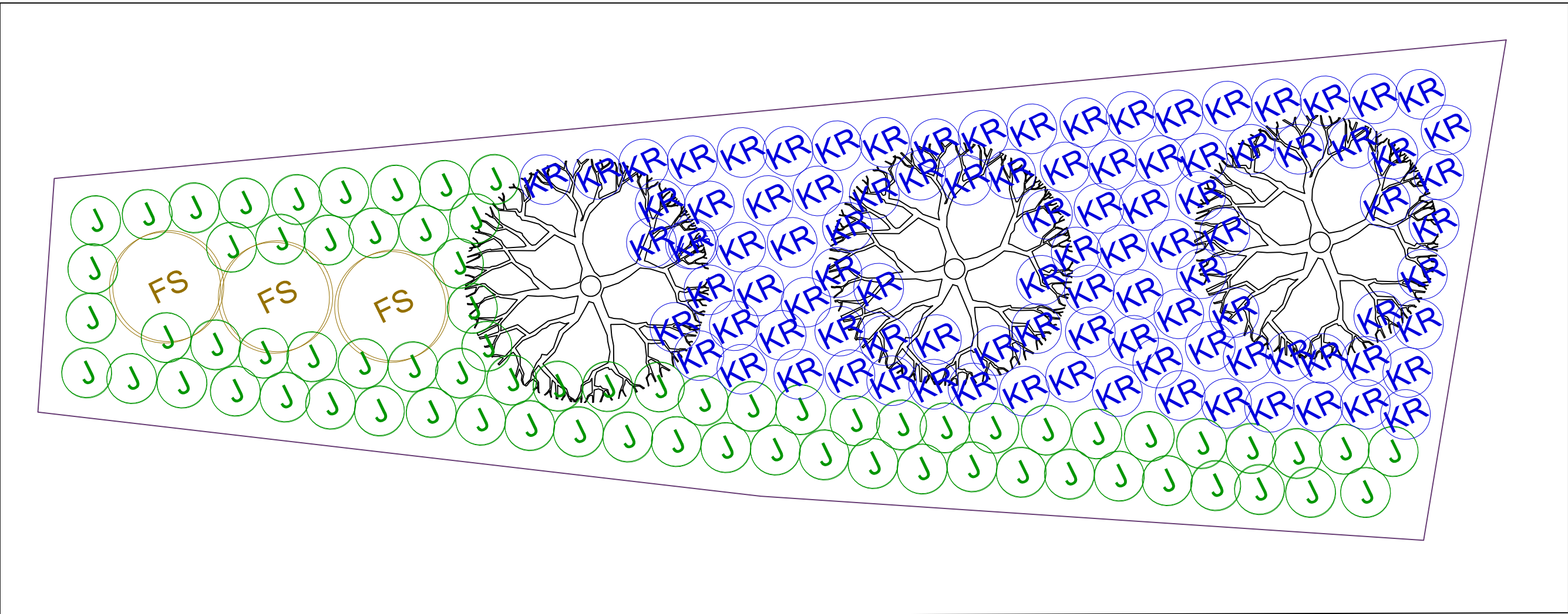
Plöntuplan - beð 16 1:50
