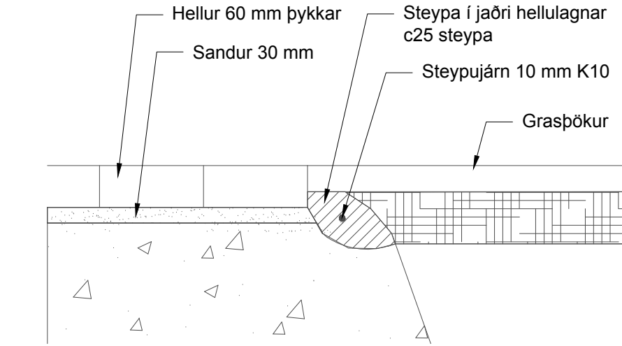
Steypa með fram hellulögn 1:10
