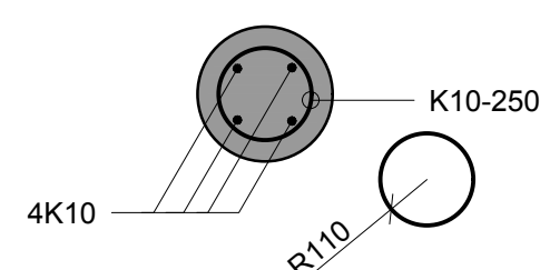
Undirstaða timbur hljóðveggs - deili 1:20
