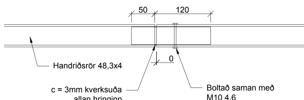
Tenging röra á handriði 1:5
