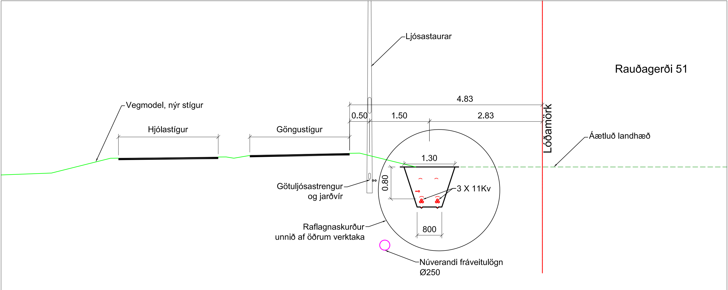
B Snið 1:50
