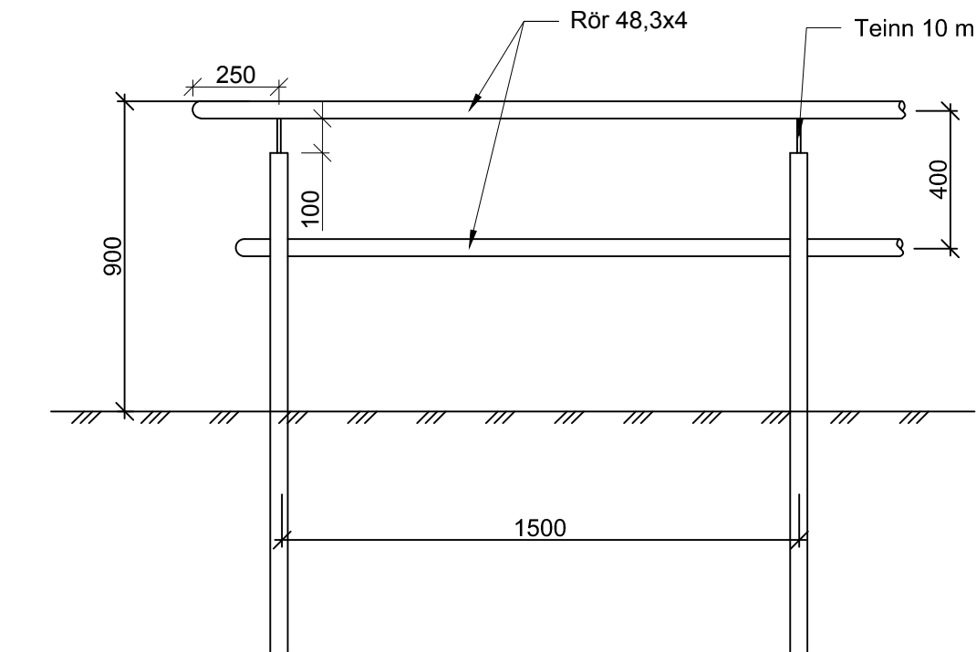
Handrið við útsýnispall - snið 1:20
