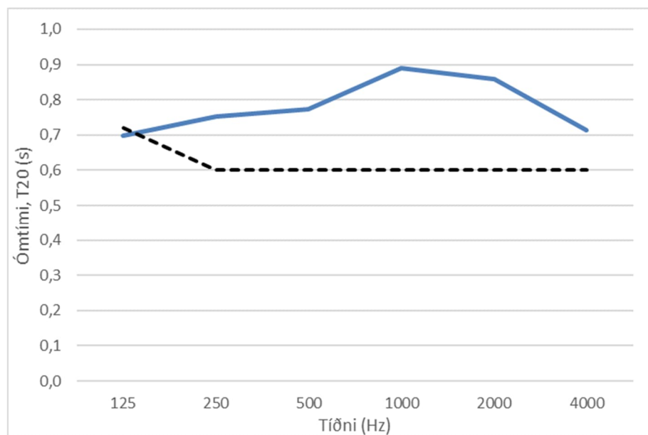
Mynd 3 Mældur ómtími og æskilegt viðmiðunargildi.
