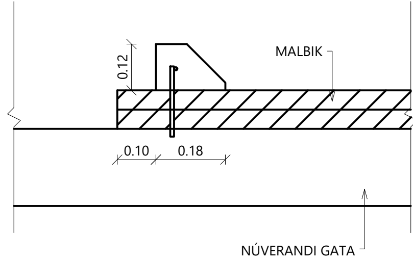
KANTSTEINN 1:10
