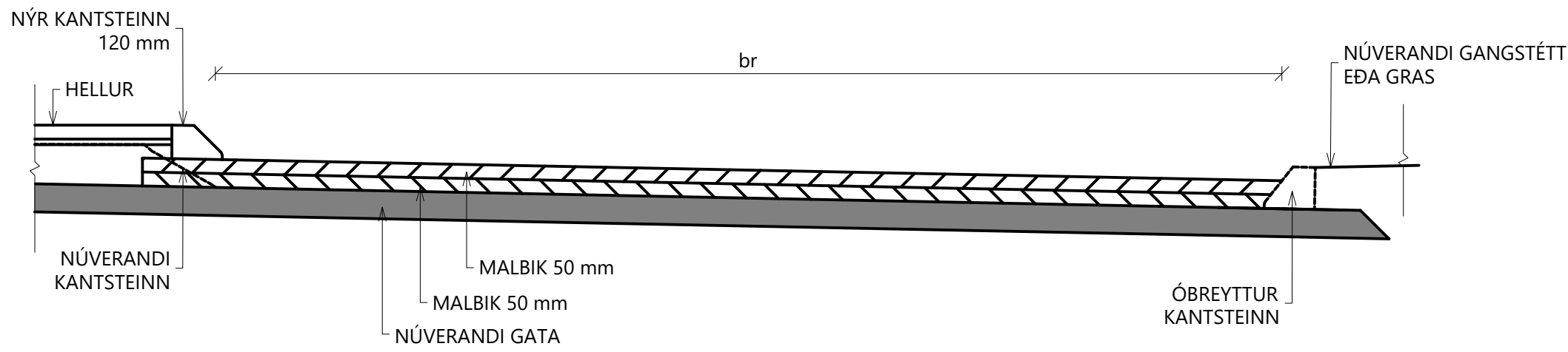
UPPHÆKKUN - KENNISNIÐ 1:20
