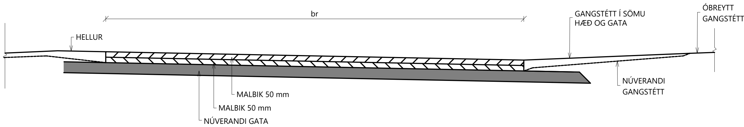
KENNISNIÐ Í UPPHÆKKAÐRI GANGBRAUT 1:20
