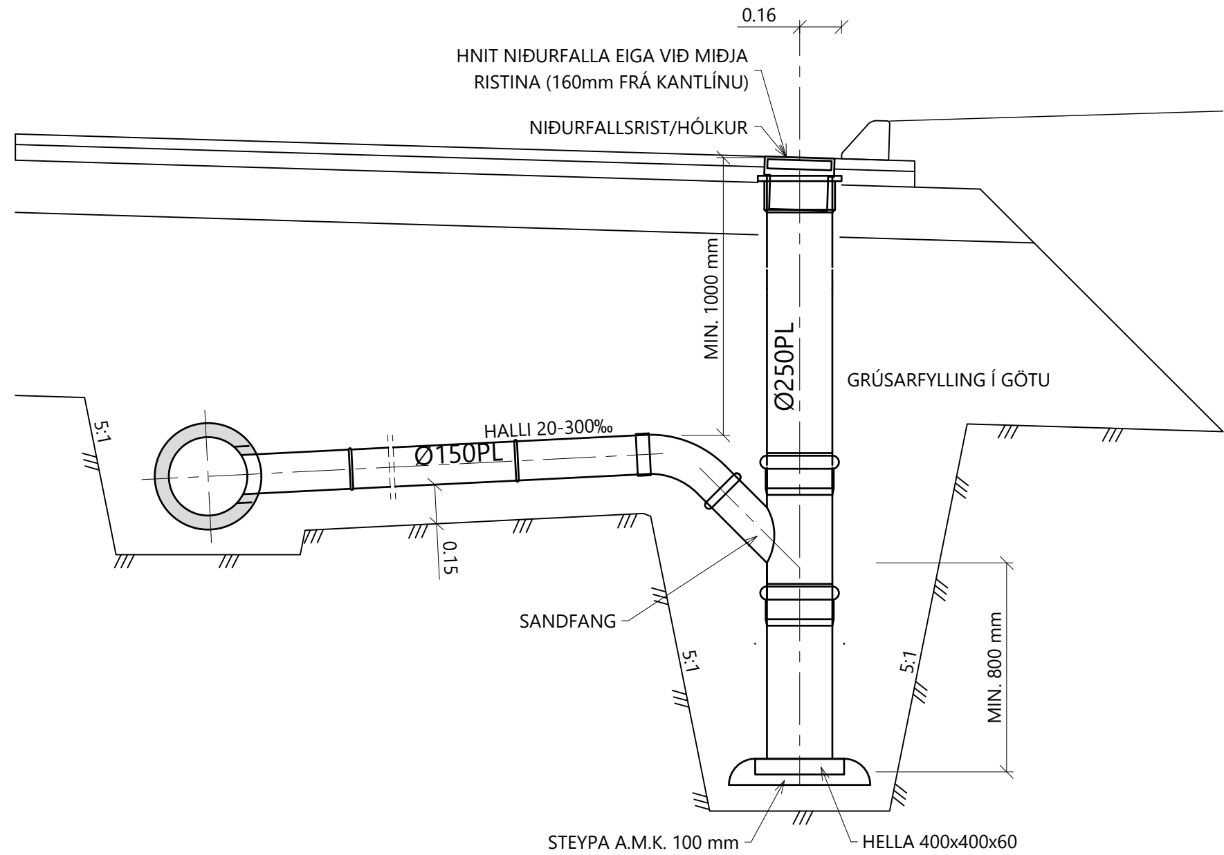
NIÐURFALL - FRÁGANGUR 1:20
