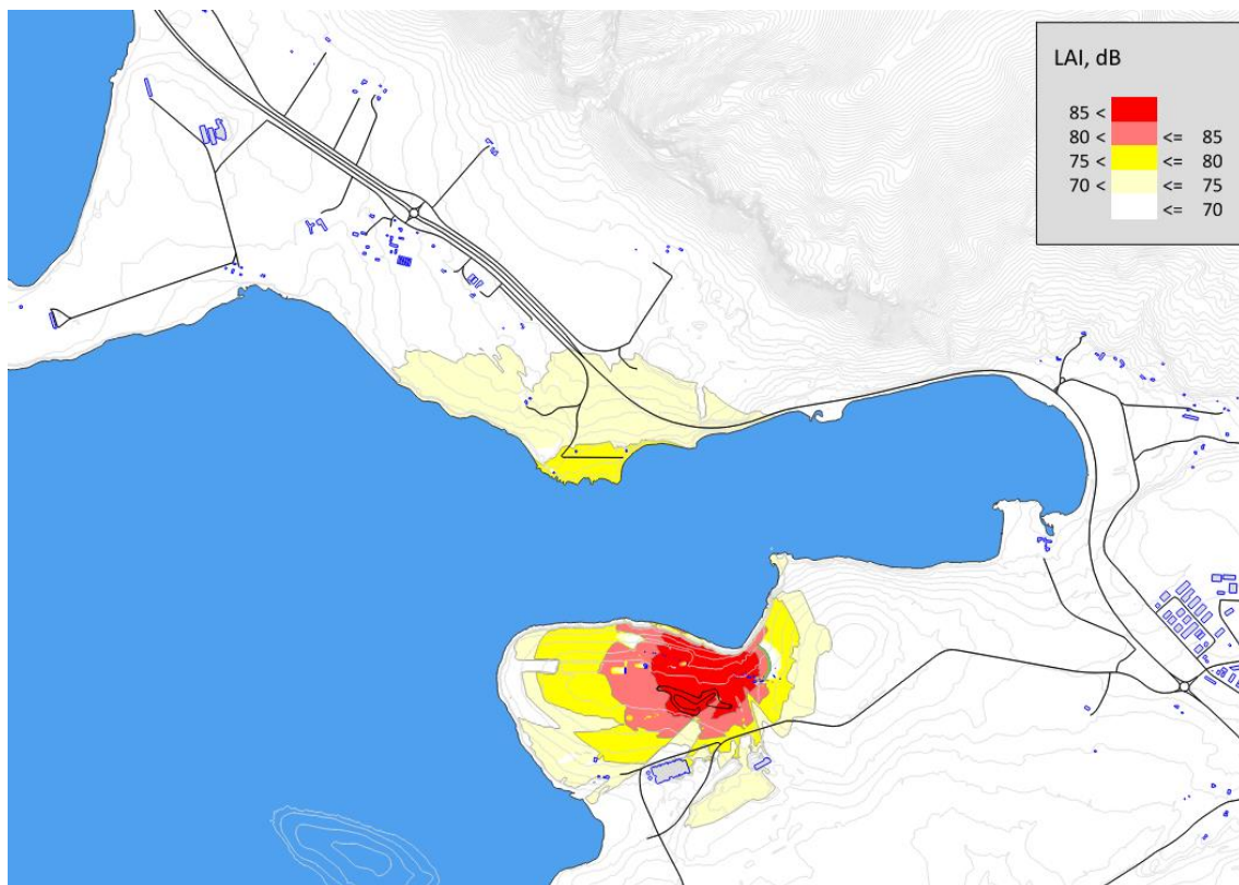
Mynd 7 Völlur 1 eingöngu með höfuðskotstefnu snúið í vestur. Reiknað augnabliksgildi, frísviðsgildi í 1,5 m hæð, L_{AI} (dB).
