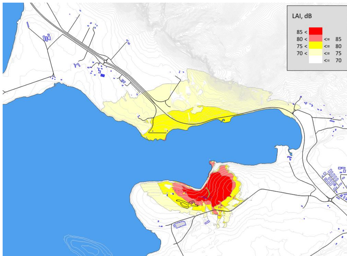
Mynd 5 Reiknað augnabliksgildi, frísviðsgildi í 1,5 m hæð, L_{A1} (dB). Hávaði frá öllum völlum.
