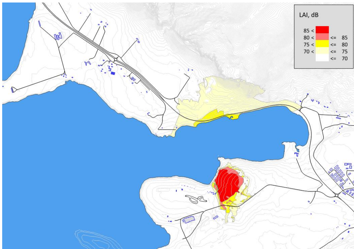
Mynd 6 Völlum 4 eingöngu. Reiknað augnabliksgildi, frísviðsgildi í 1,5 m hæð, L_{A1r} (dB).
