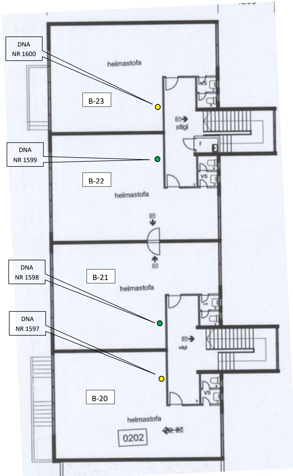
Mynd 1: Grunnmynd 2. hæð B - álmu.
