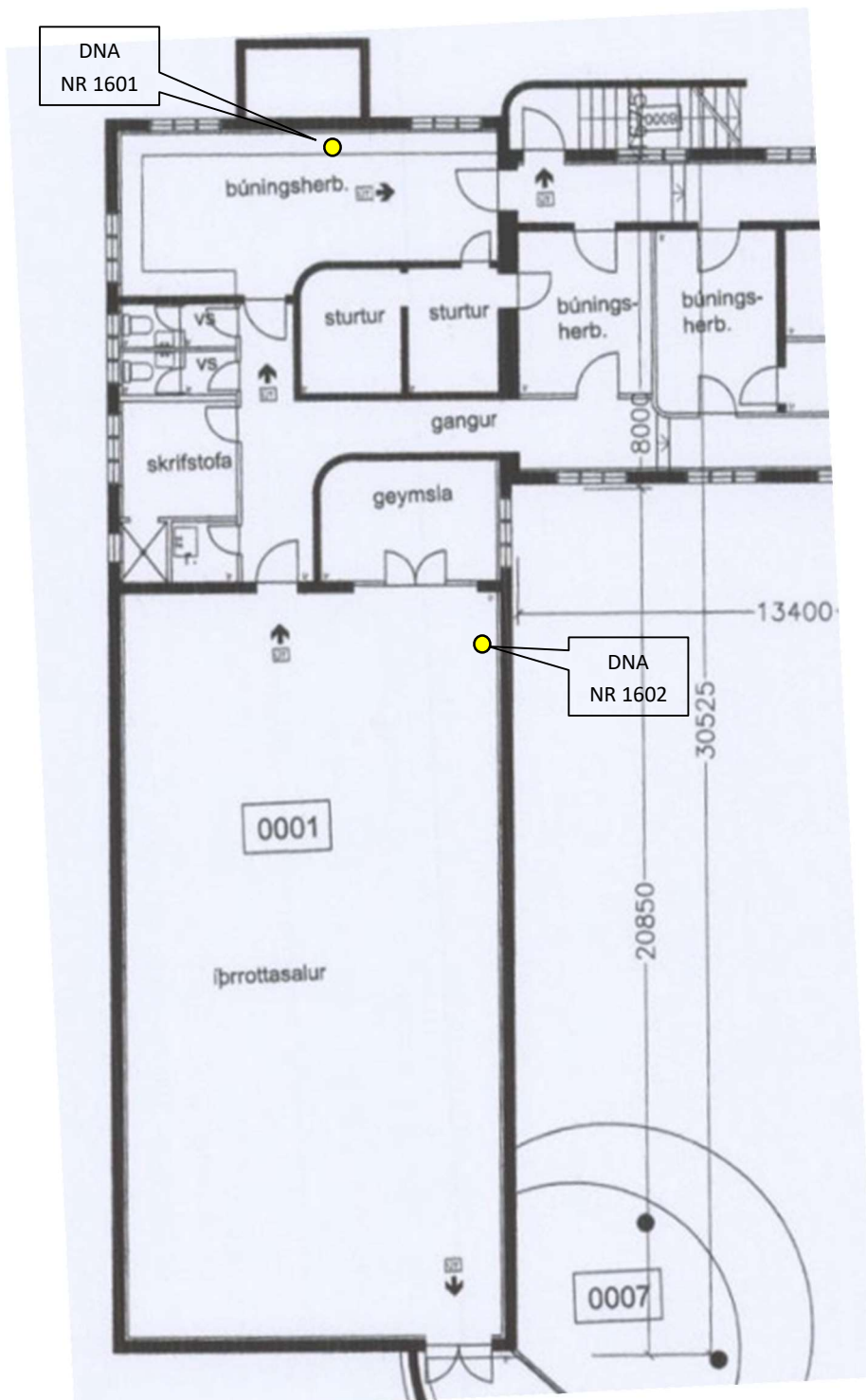
Mynd 2: Grunnmynd Íþróttahúss, kjallari.
