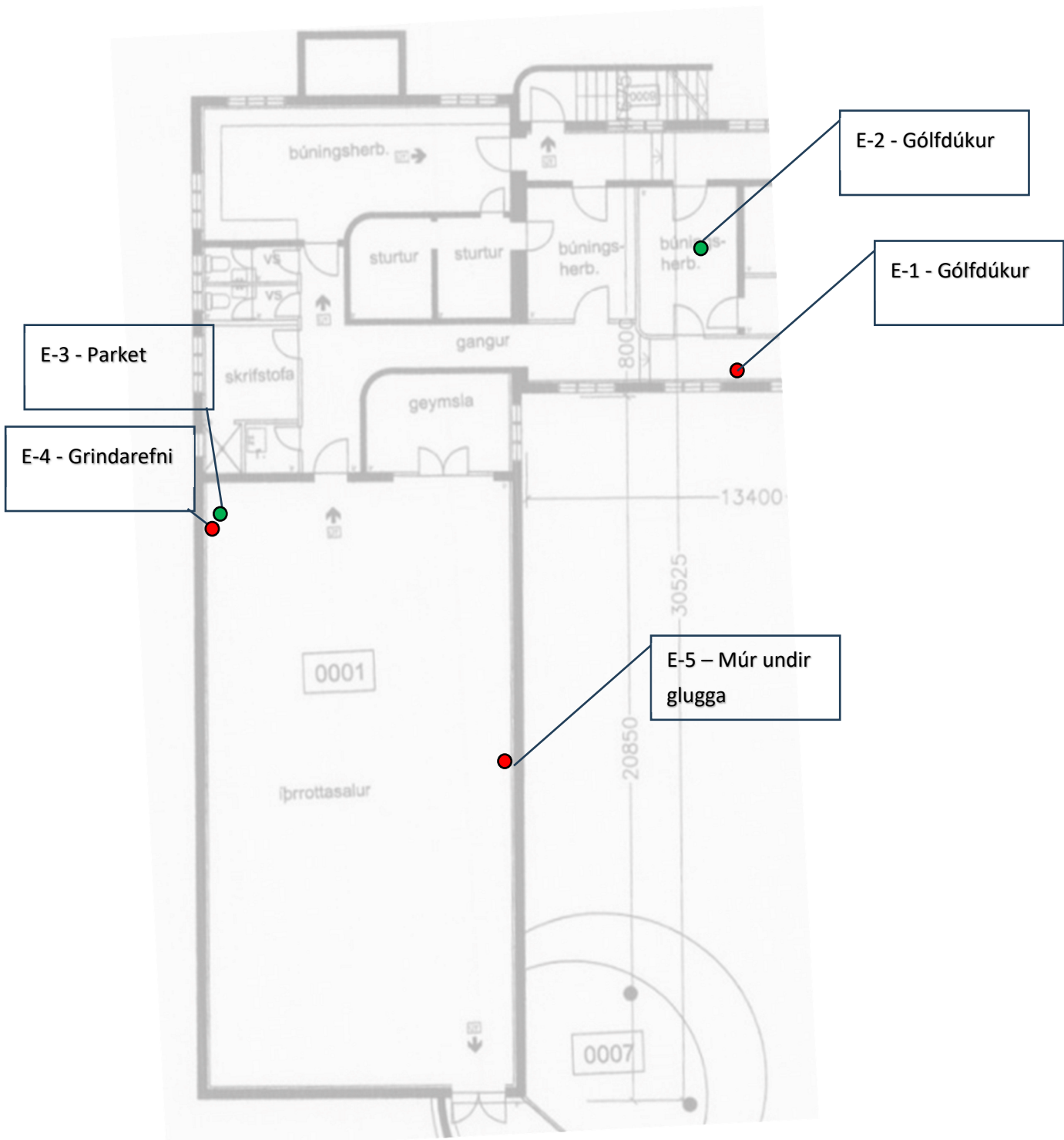
Mynd 1: Grunnmynd Íþróttahúss, kjallari.
