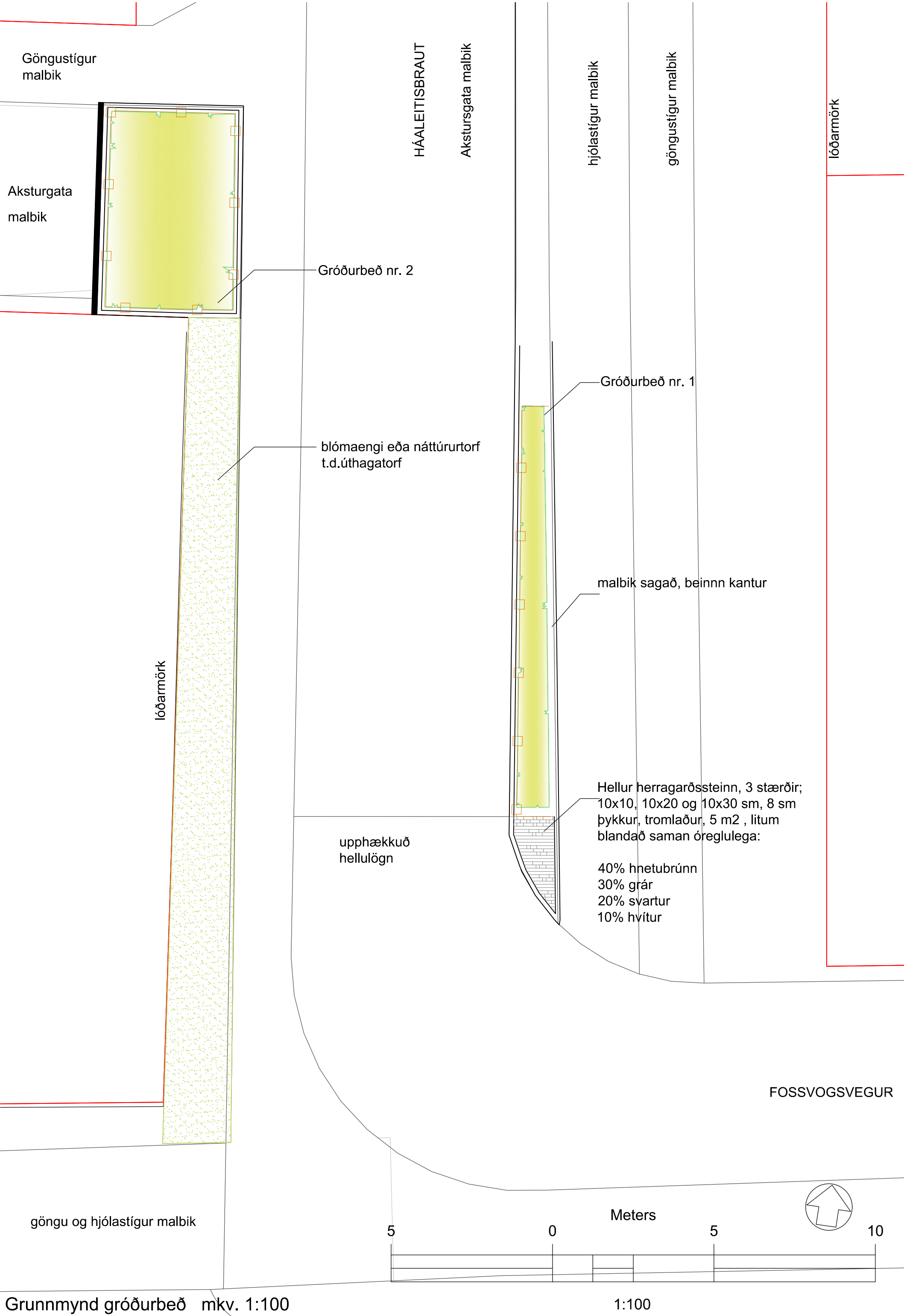
Grunnmynd gróðurbeð mkv. 1:100
