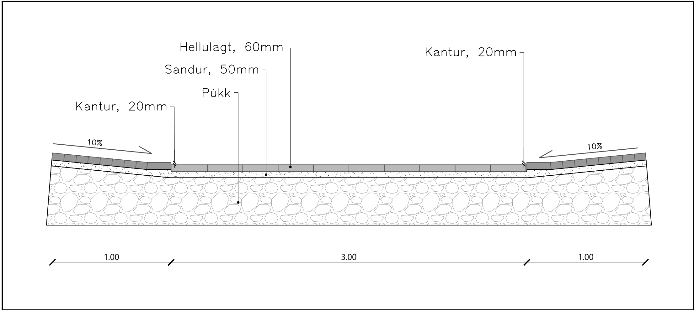
Miðeyja gangbrautar, 1:20
