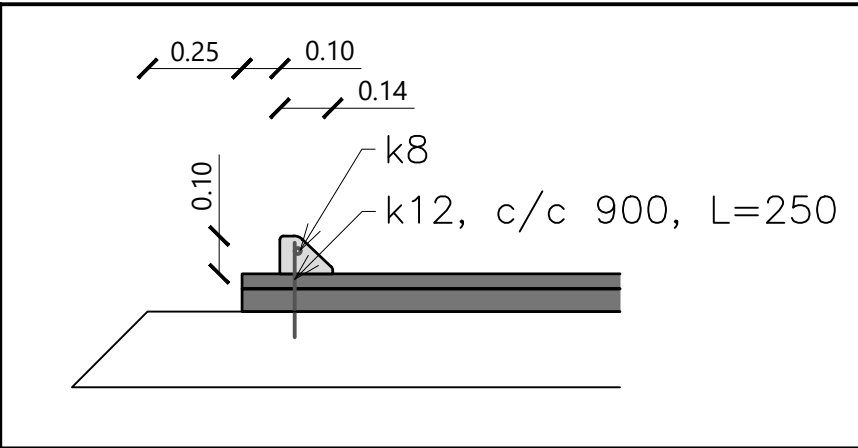
Kantsteinn, 1:20
