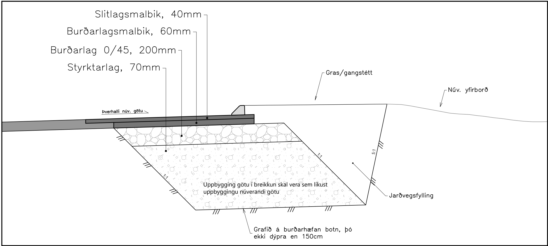
Breikkun götu, 1:20
