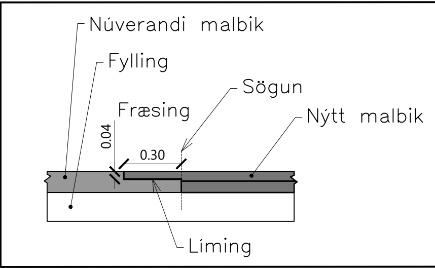
Fræstur lás, 1:20
