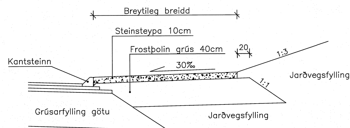
ÞVERSNIÐ ÞAR SEM LÓÐ ER HÆRRI EN STÉTT
