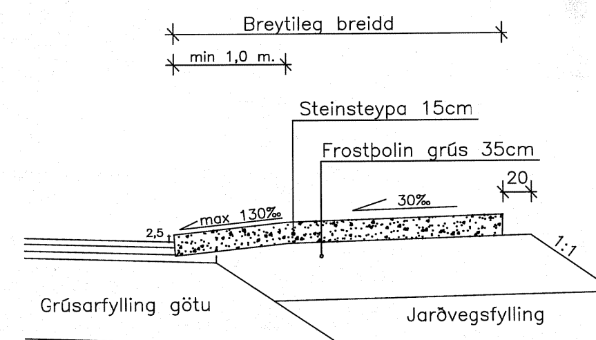
ÞVERSNIÐ INNKEYRSLU
