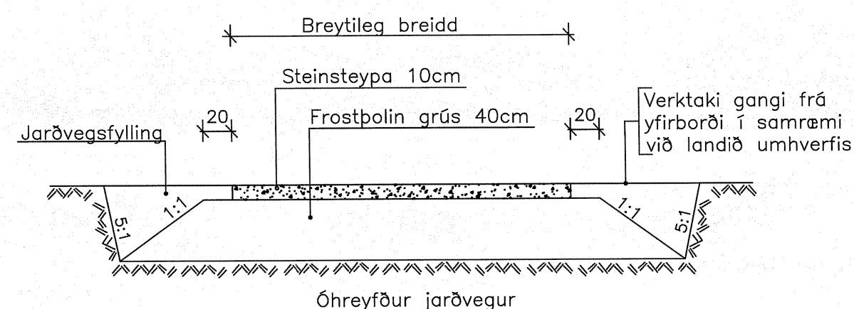
ÞVERSNIÐ GANGSTÉTTAR Í GRASEYJU
