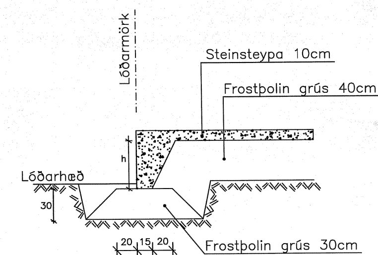
ÞVERSNIÐ, BAKKANTUR
