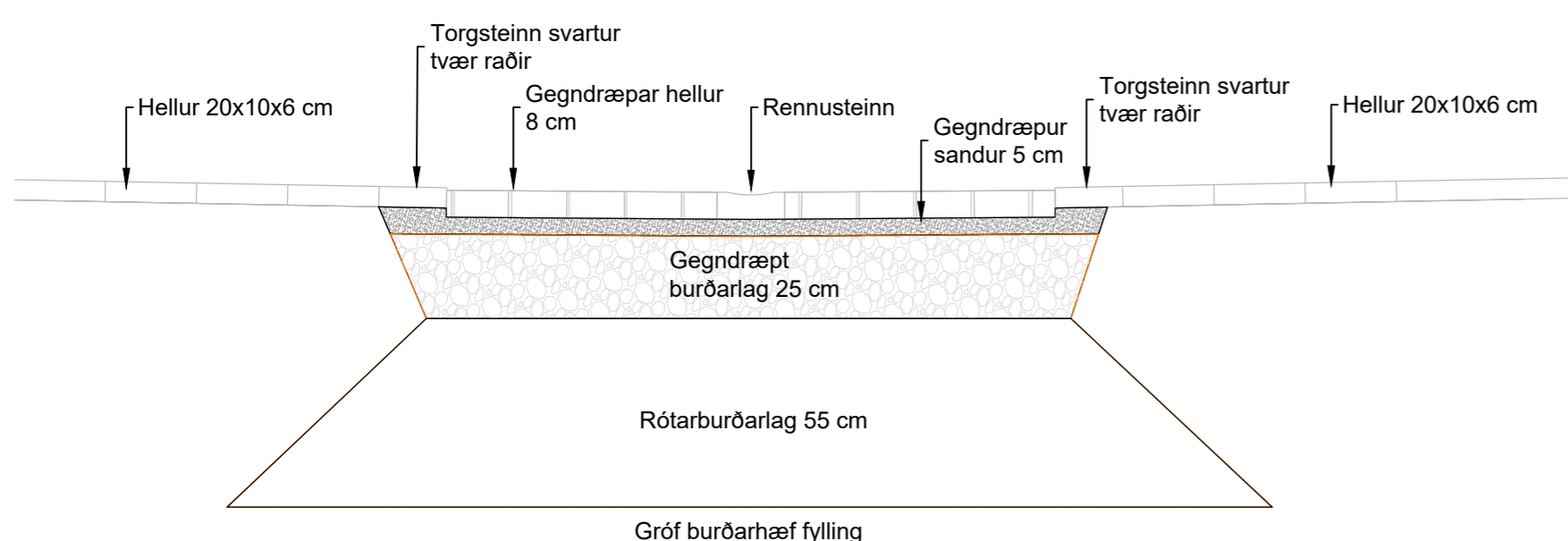
- SNIÐ Í GEGNDRÆPAR HELLUR Í OFANVATNSRÁS - 1:20
