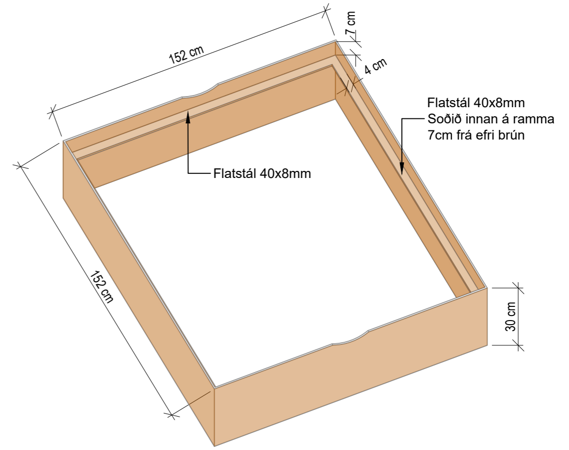
- STÁLRAMMI FYRIR STÖK GÖTUTRÉ - 1:20
