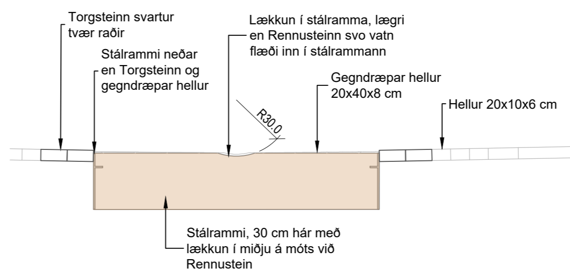
- SNIÐ - STÁLRAMMI Í OFANVATNSRÁS - 1:20
