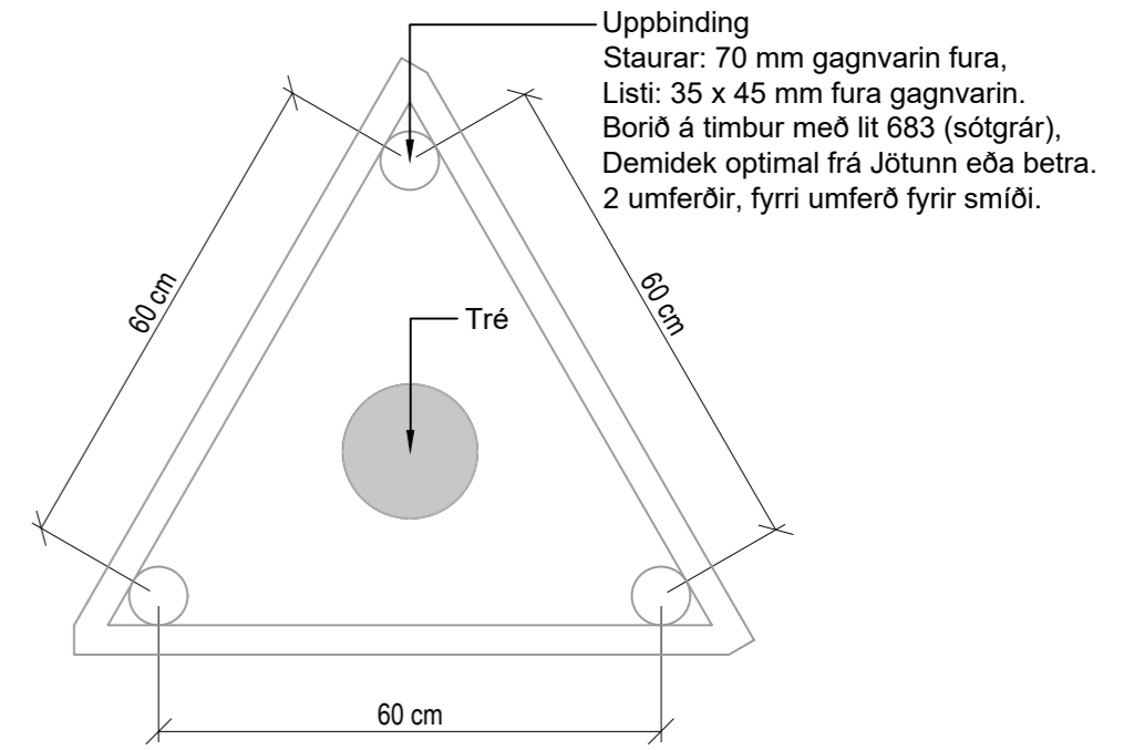
- UPPBINDING Í TRÉ - 1:10
