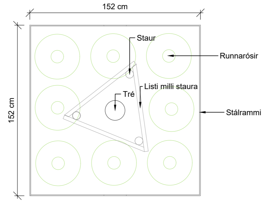
- GRUNNMYND - STÁLRAMMI OG UPPBINDING - 1:20
