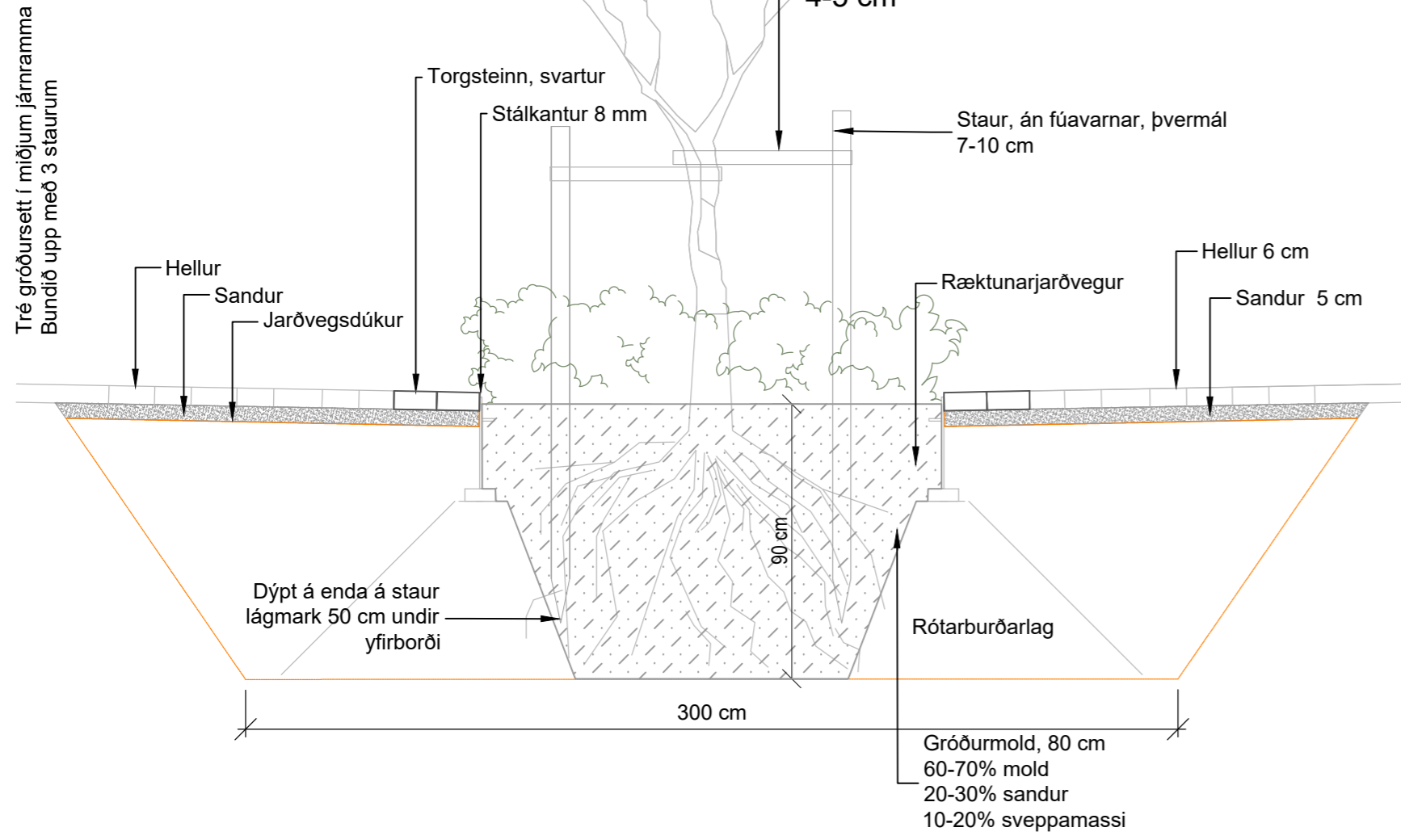
- SNIÐ - UPPBINDING TRÉ - 1:20
