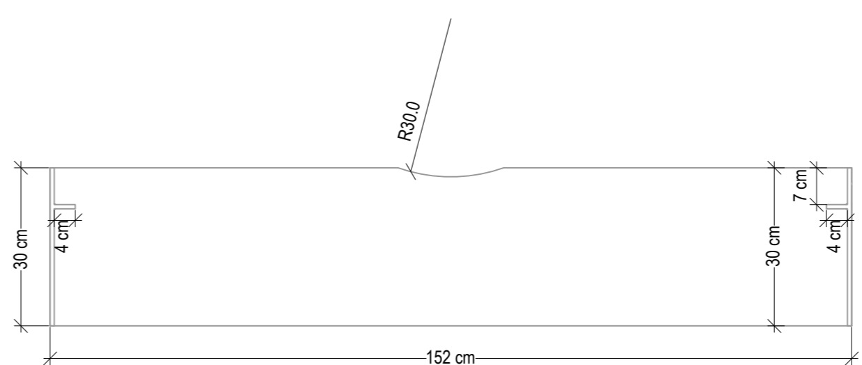
- SNIÐ - FLATSTÁL SOÐIÐ INNAN Á RAMMA - 1:10
