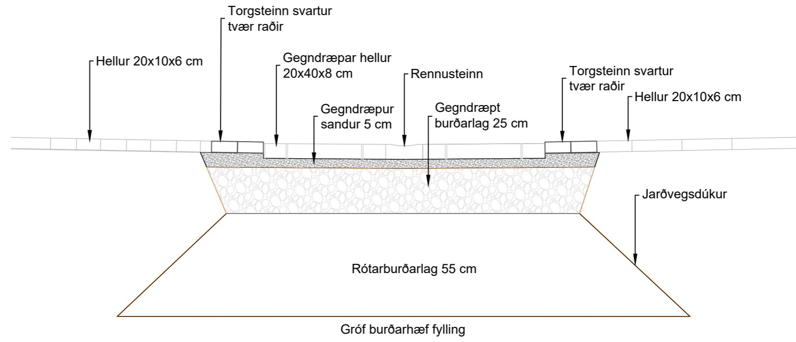
- SNIÐ - OFANVATNSRÁS, SVÆÐI MILLI TRJÁRAMMA - 1:20
