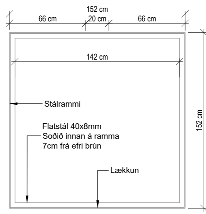
- STÁLRAMMI FYRIR STÖK GÖTUTRÉ - 1:20
