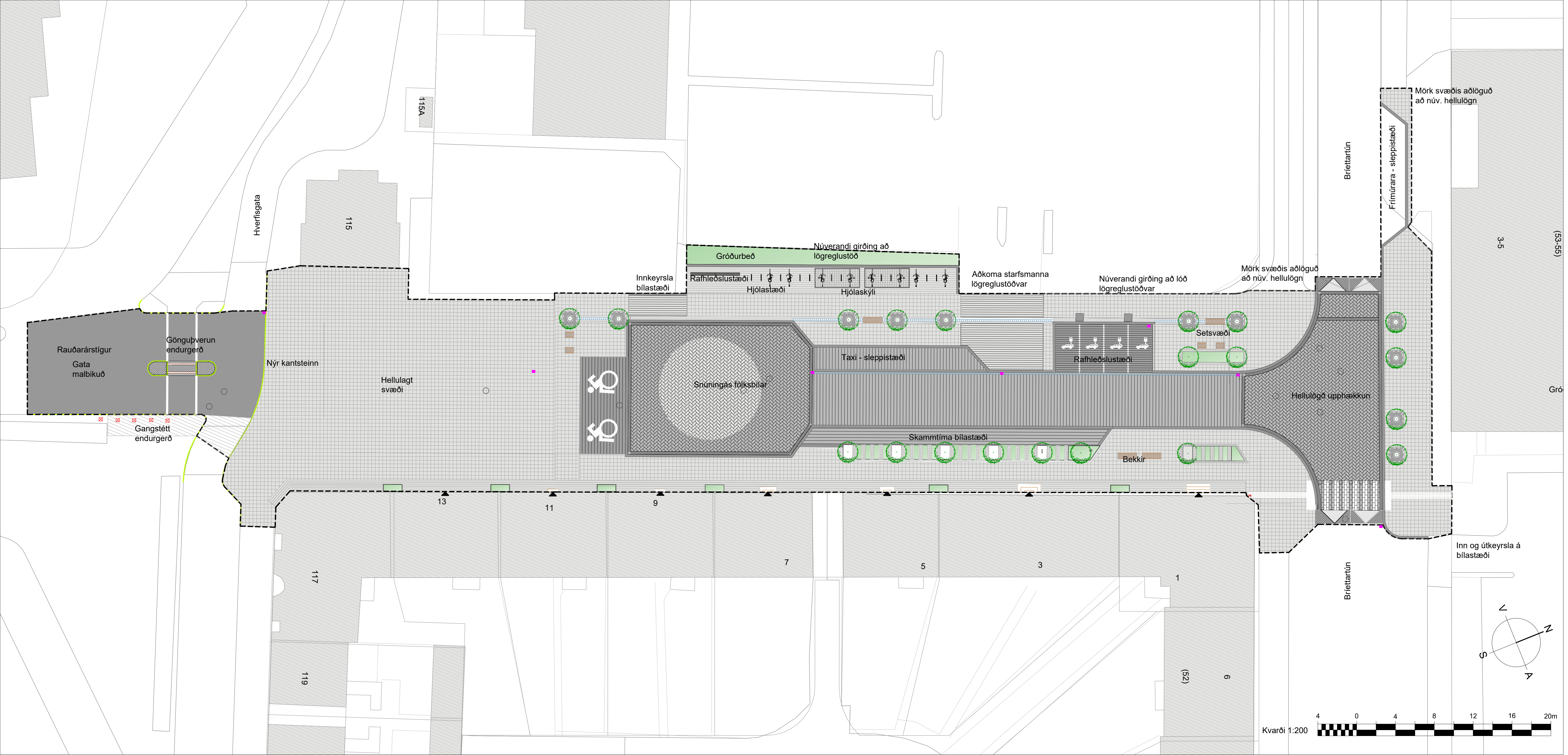
Grunnmynd, 1:200
