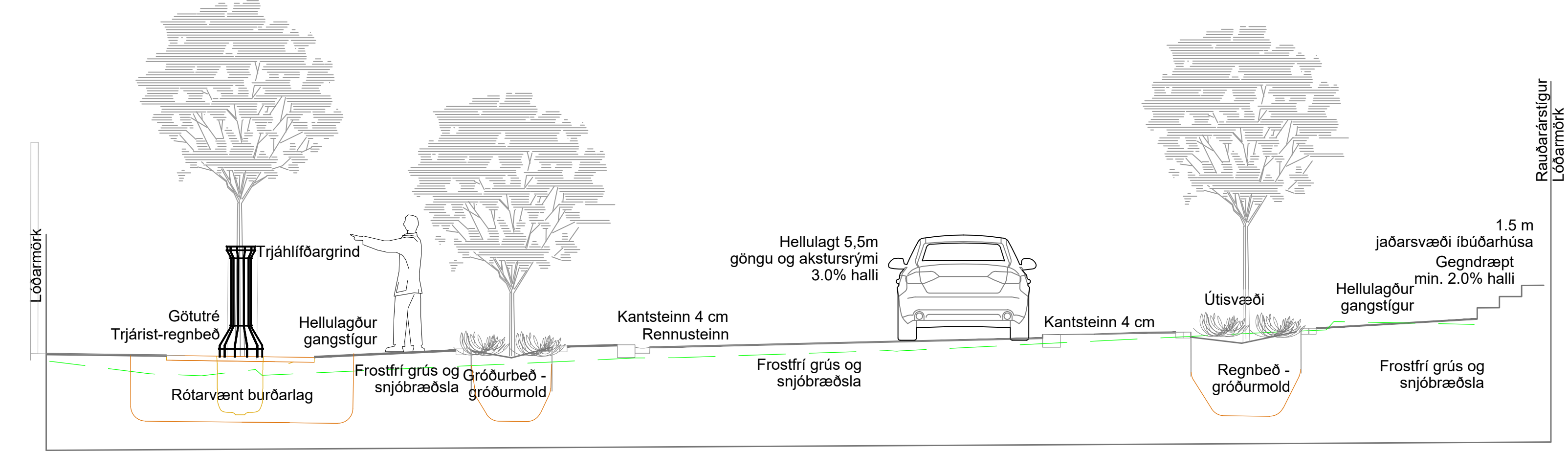
1 Snið 1:50 LL-F-G-01
