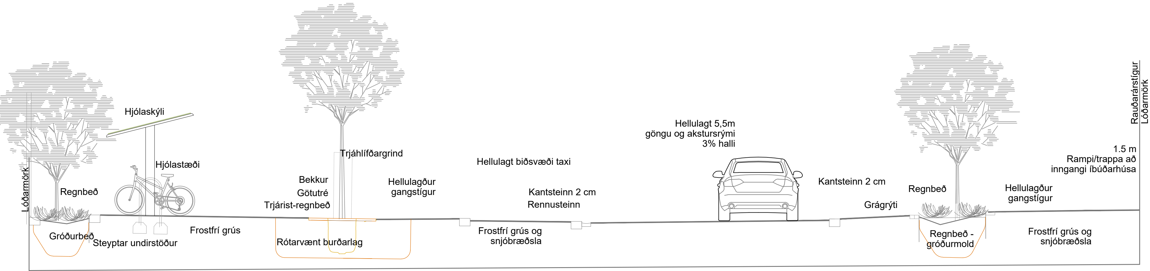
2 Snið 1:50 LL-F-G-01
