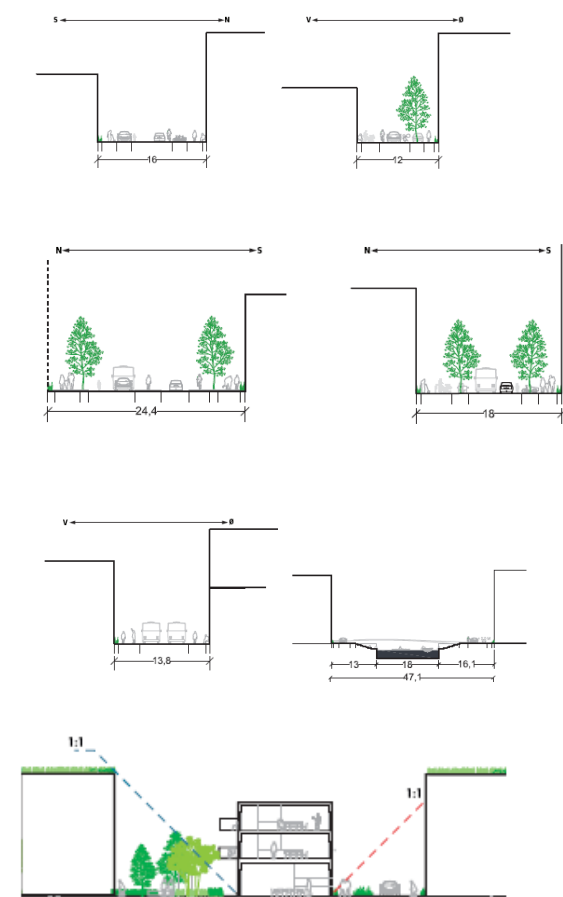
Mynd 13. Hér sjást æskileg viðmið þegar kemur að því að meta breidd gatna í hlutfalli við hæð byggðar.
