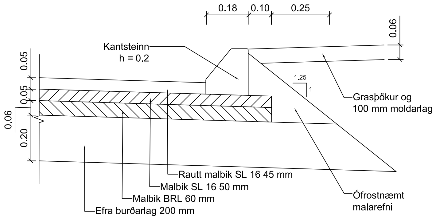
Frágangur 200 mm kantsteins við strætórein- 1:10
