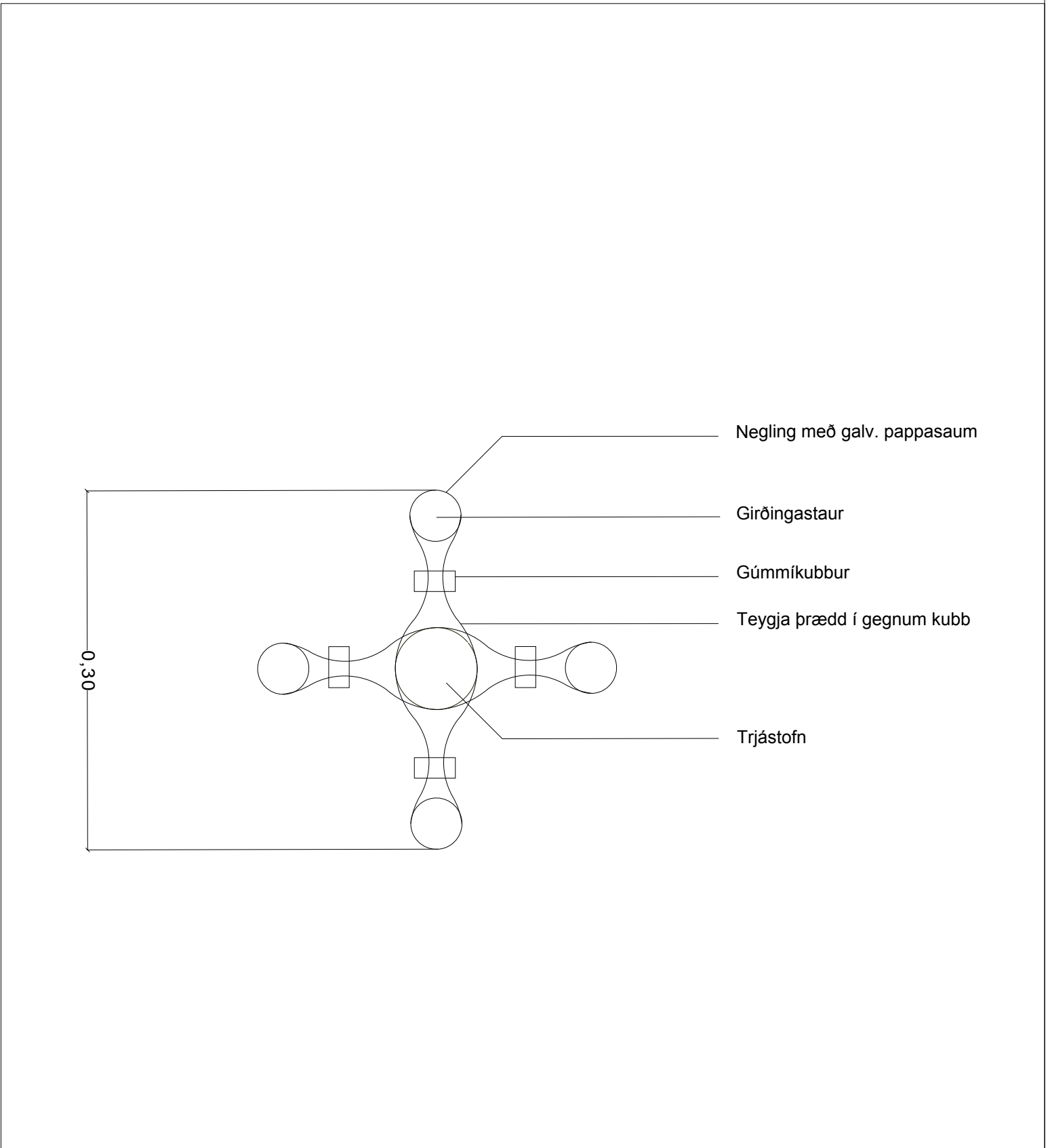
Deiliteikning 7; 1:5
