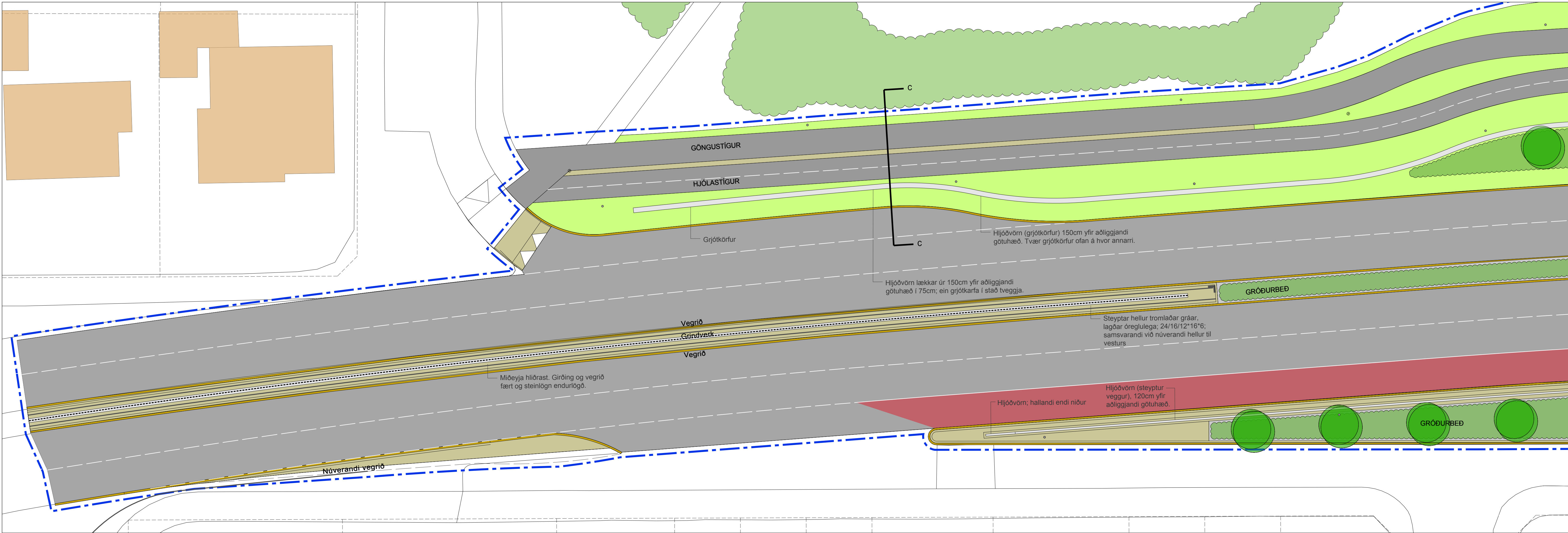
Vesturhluti 1:200
