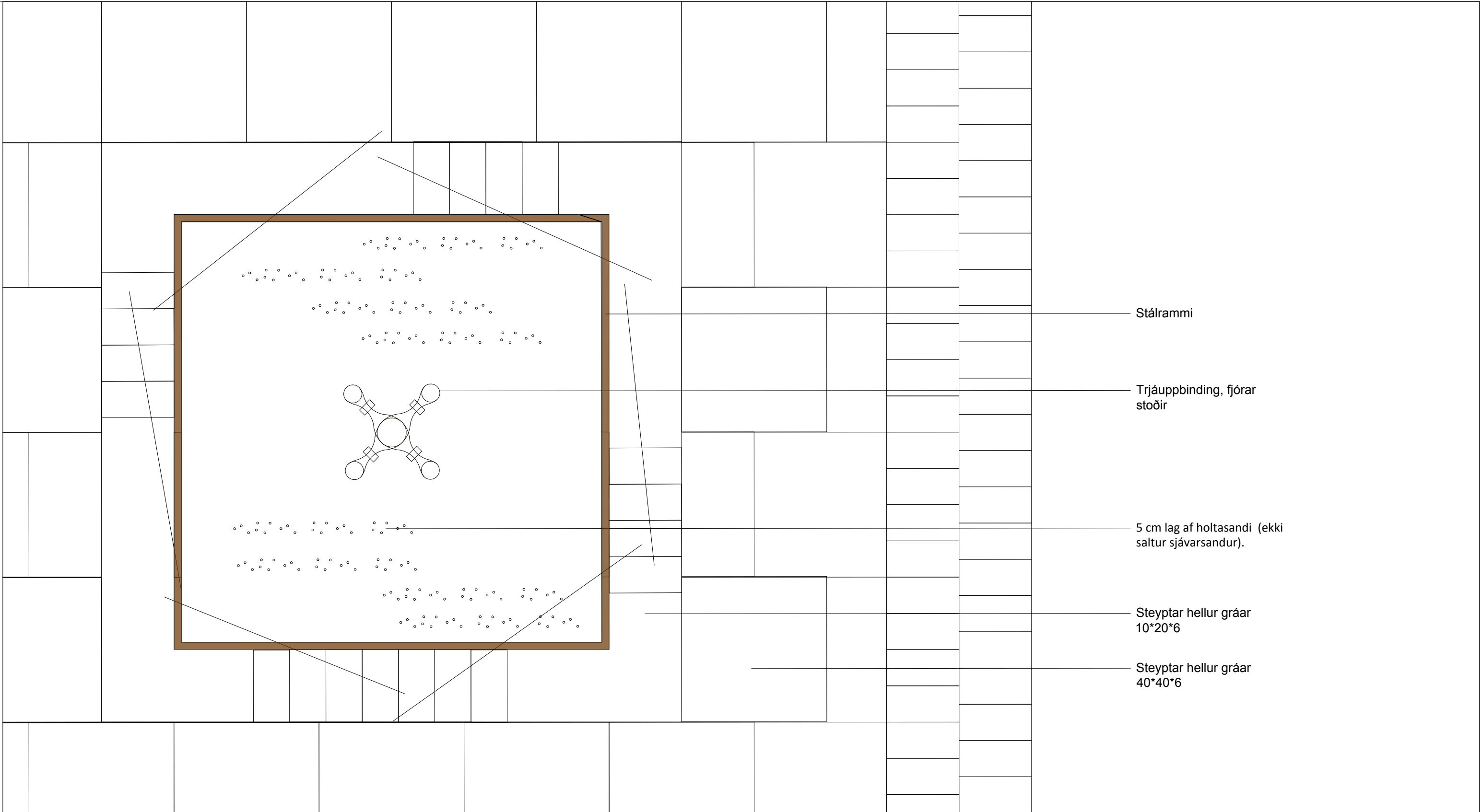
Deiliteikning 5; 1:10
