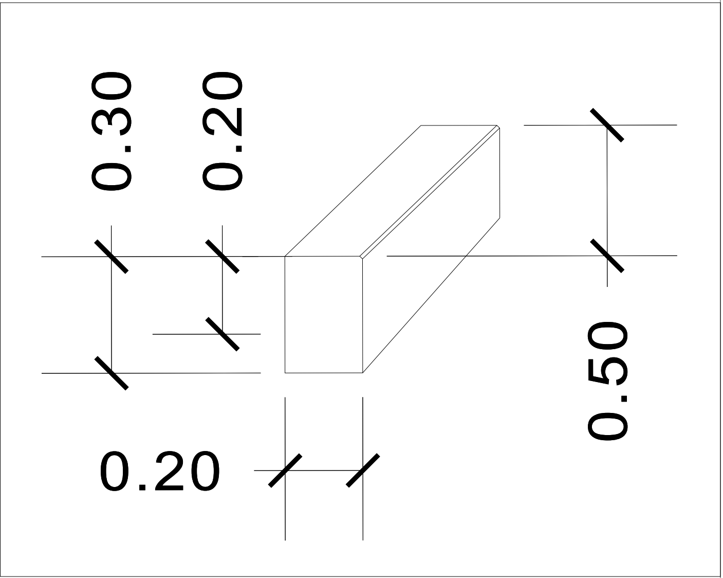
Deiliteikning 3; kantsteinn á biðstöð 1:20
