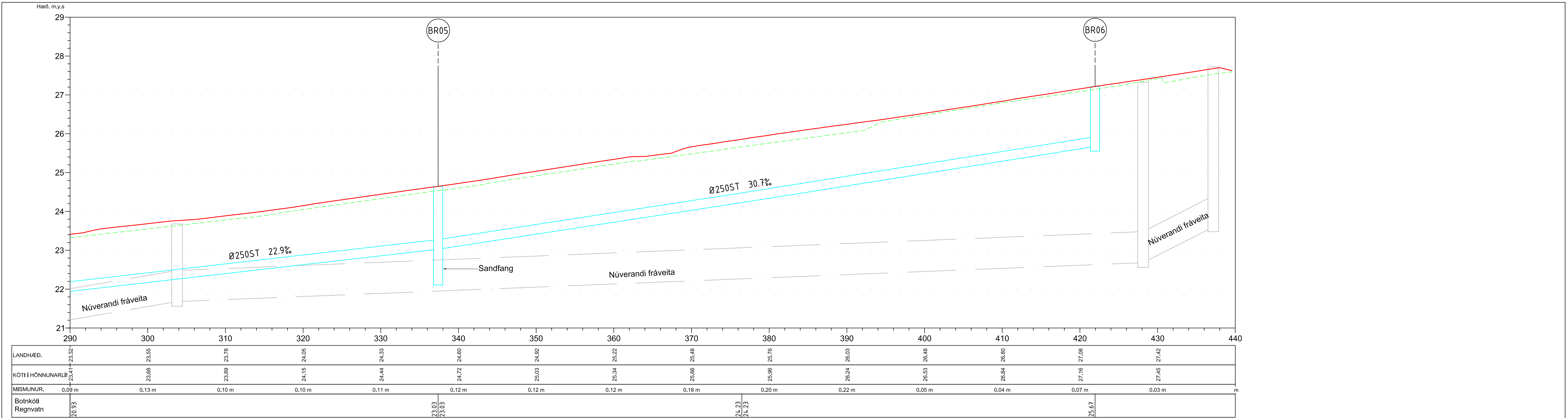
Langsnið 1:250/1:100
