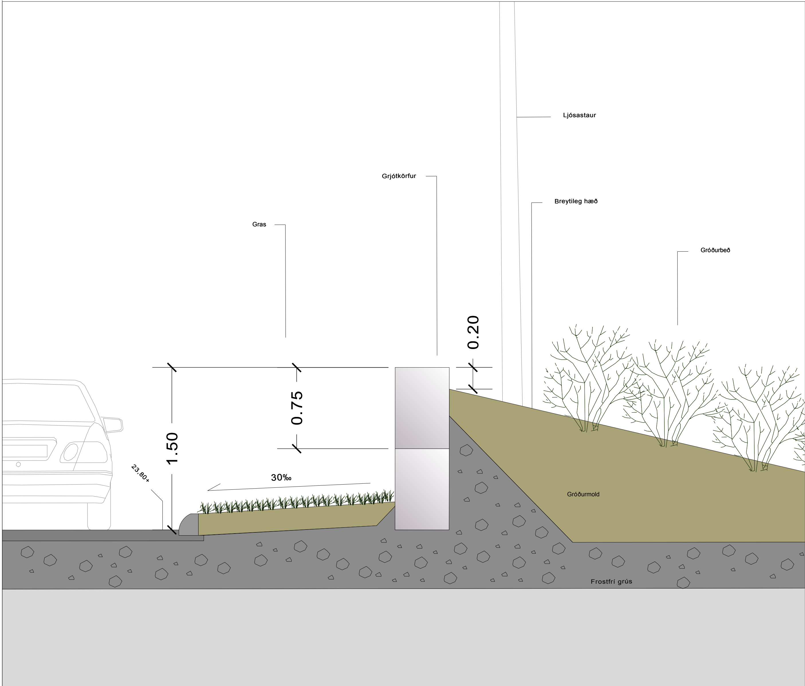
Deiliteikning 1; grjótkörfur grundun 1:20
