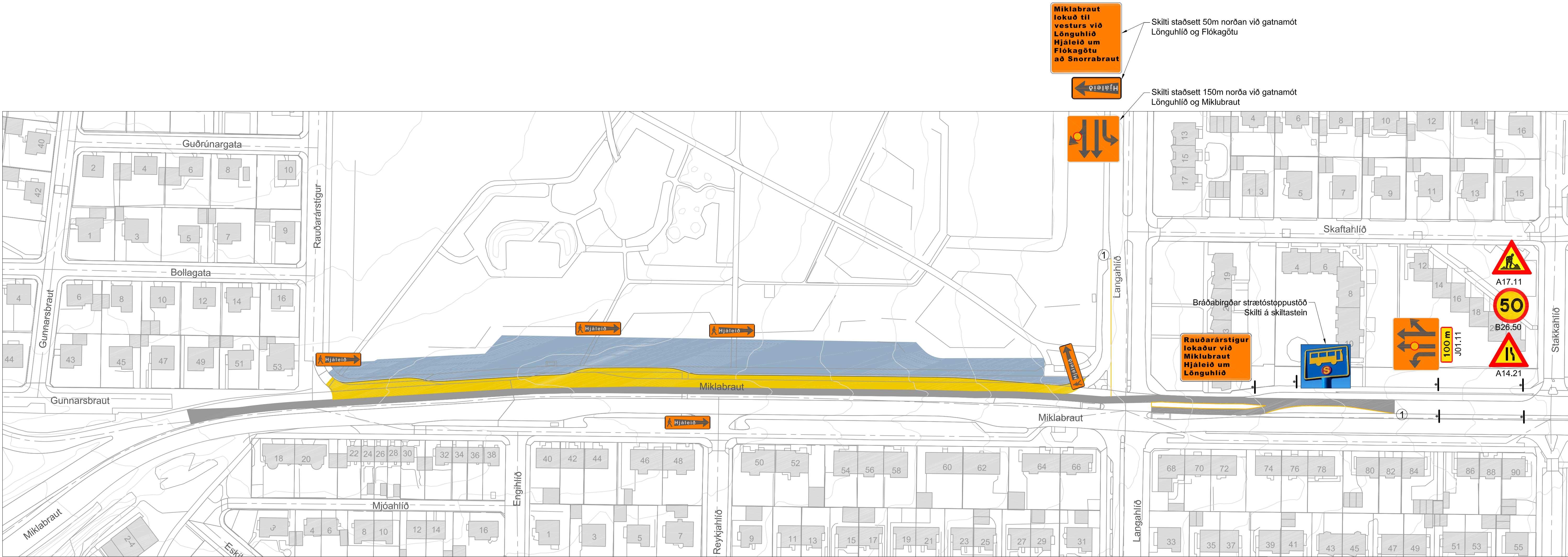
Framkvæmdasvæði 1 1:1000
