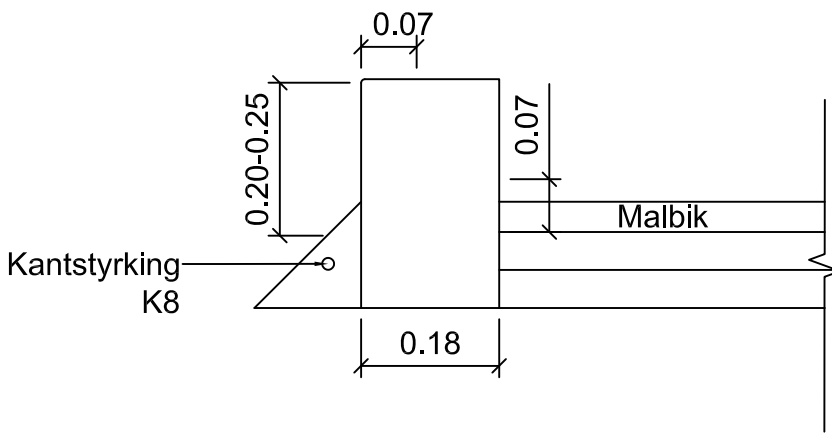
Forsteyptur kantsteinn 200 mm - 1:10
