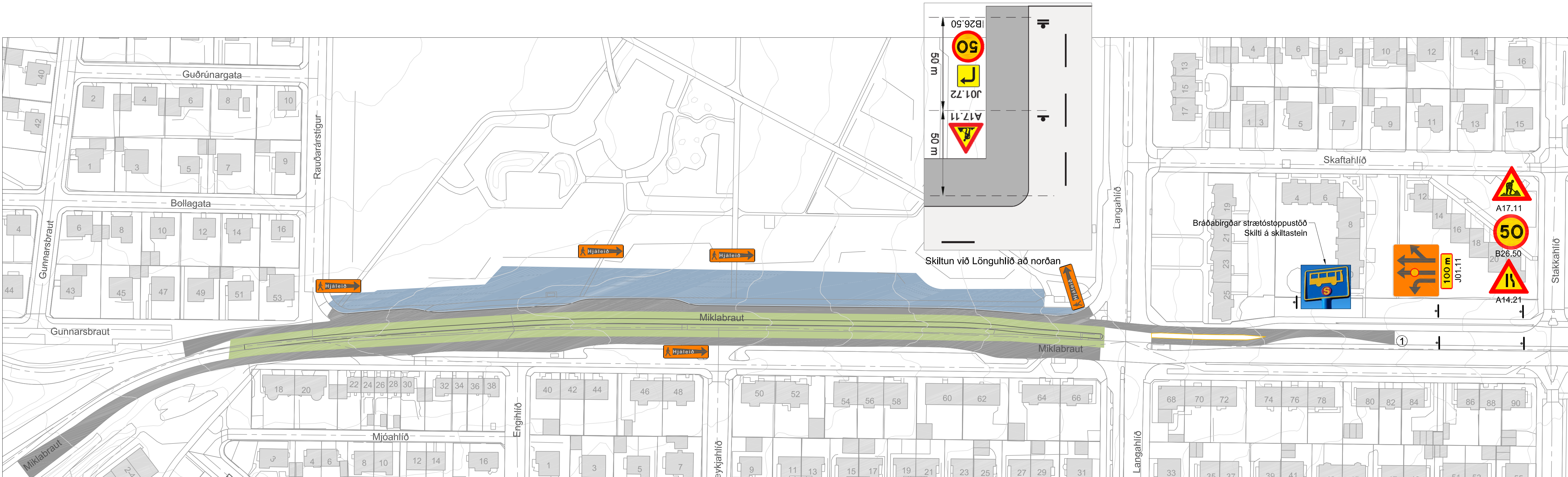
Framkvæmdasvæði 2 1:1000
