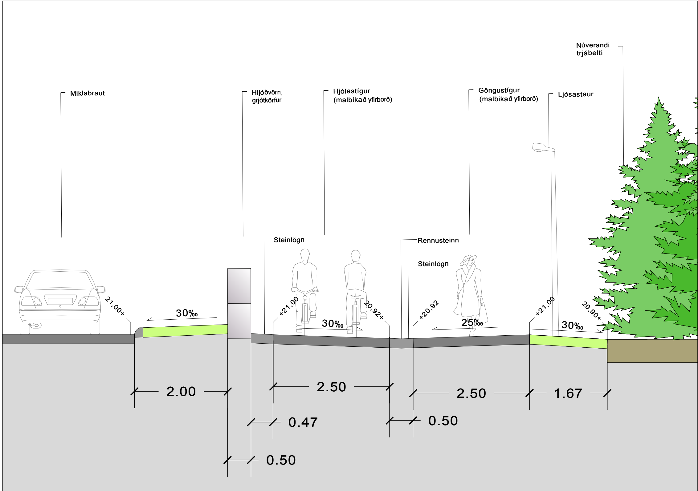
Kennisnið C-C; 0,5 m deilirými 1:50
