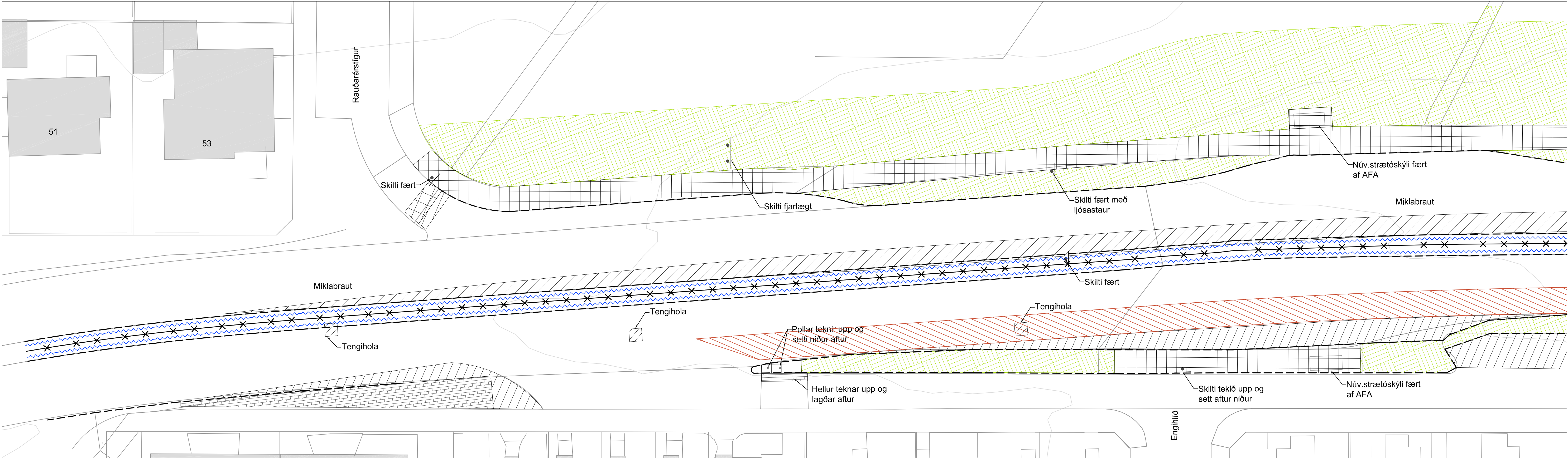
Grunnmynd 1:250
