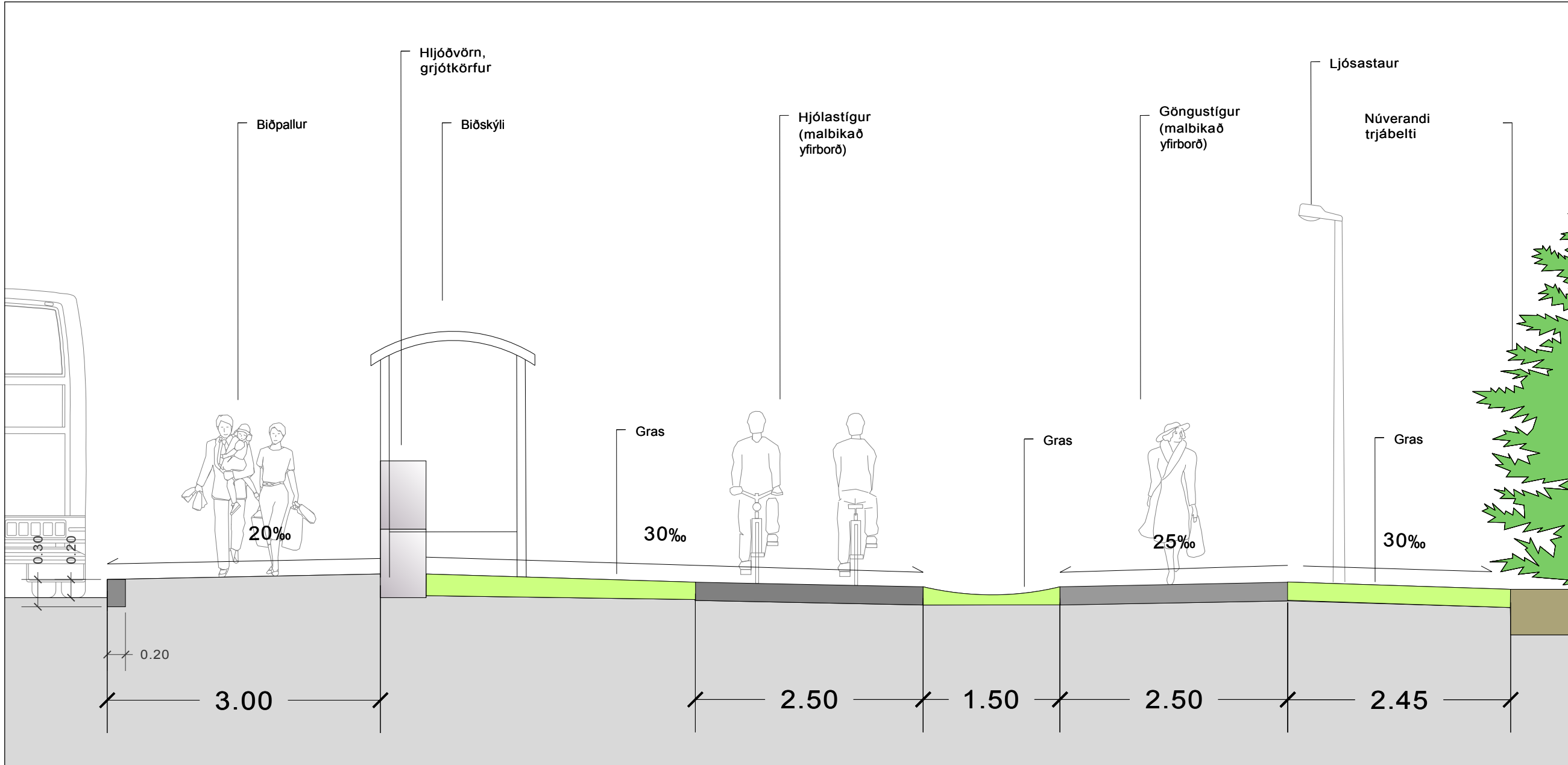
Kennisnið A-A; biðstöð við Miklatún 1:50
