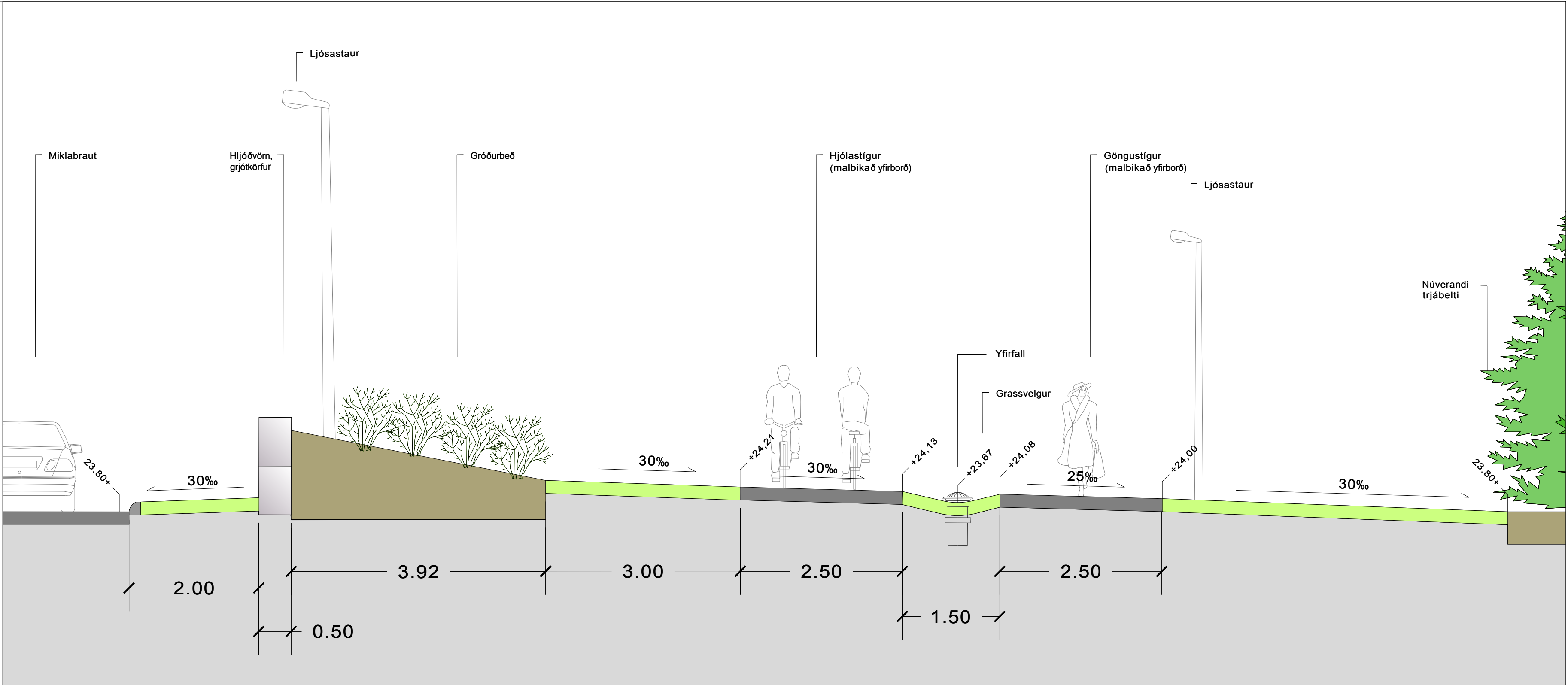
Kennisnið D-D; 1,5 m deilirými 1:50
