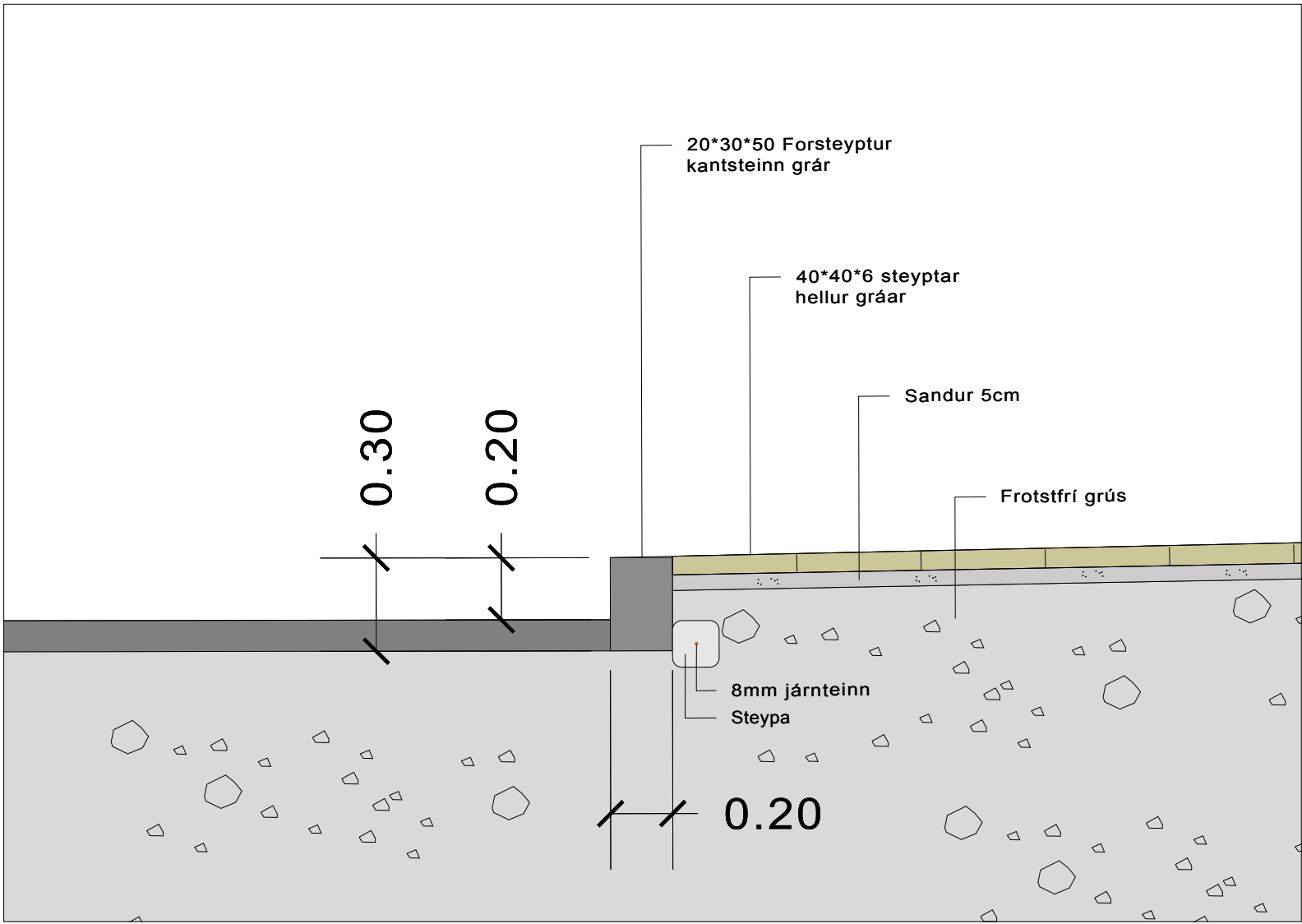
Deiliteikning 2; kantsteinn á biðstöðum 1:20
