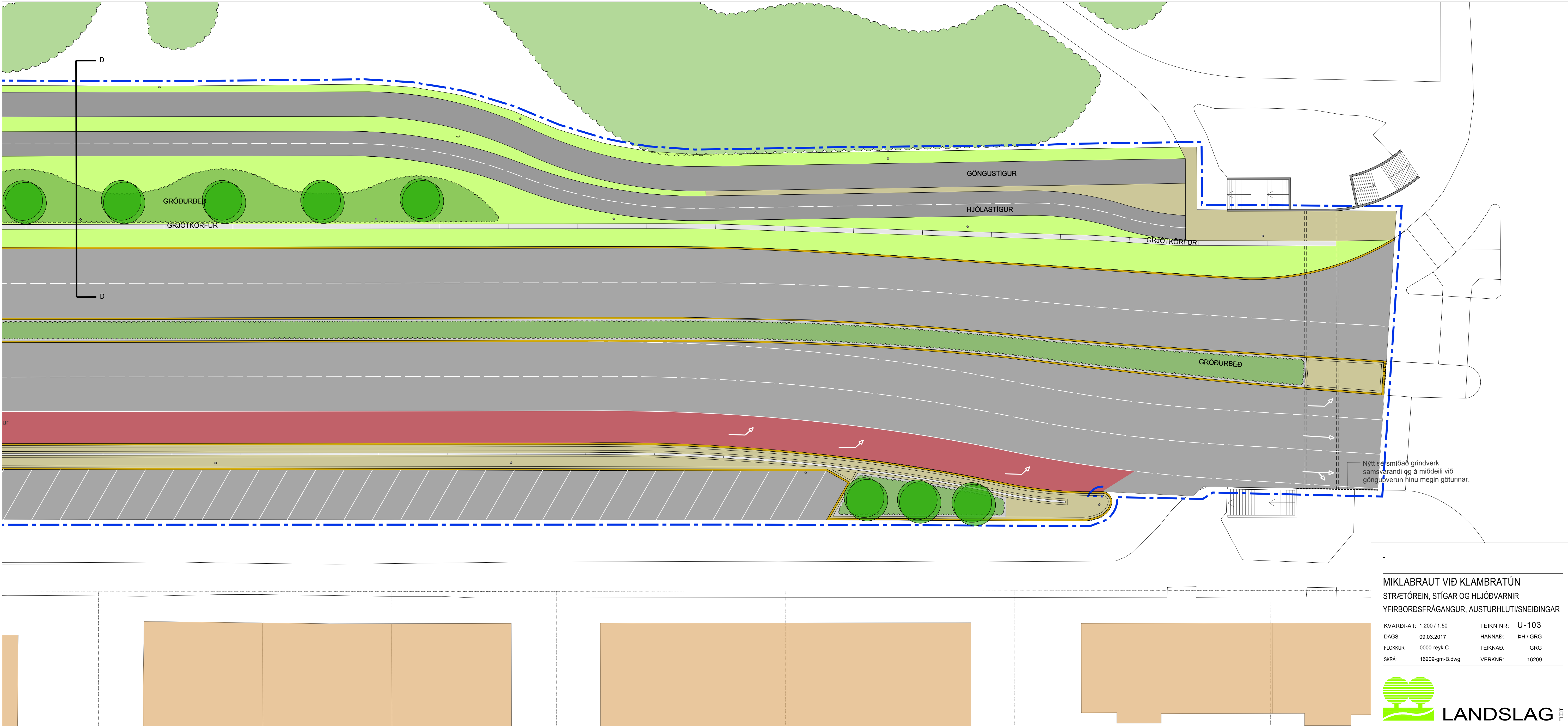
Austurhluti 1:200
