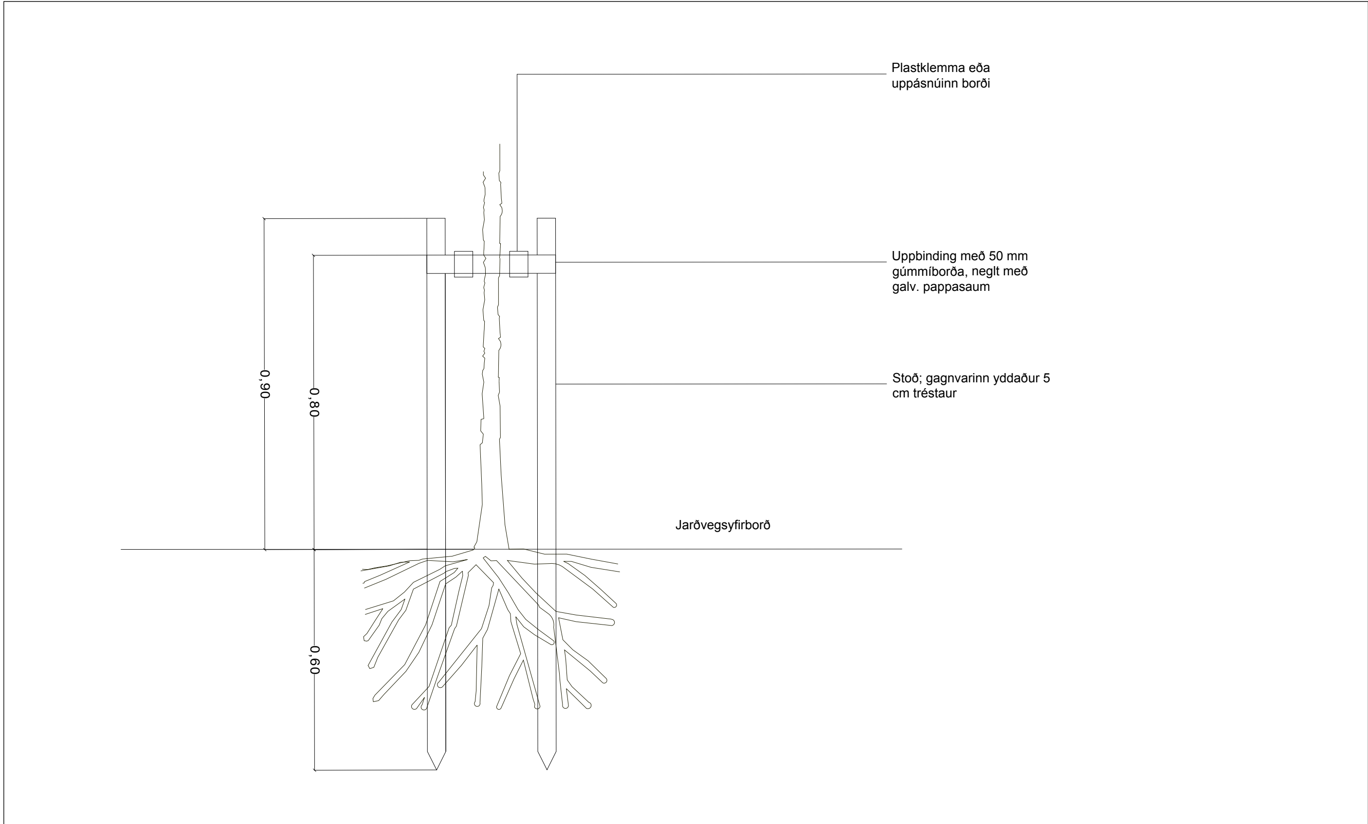
Deiliteikning 4; 1:10
