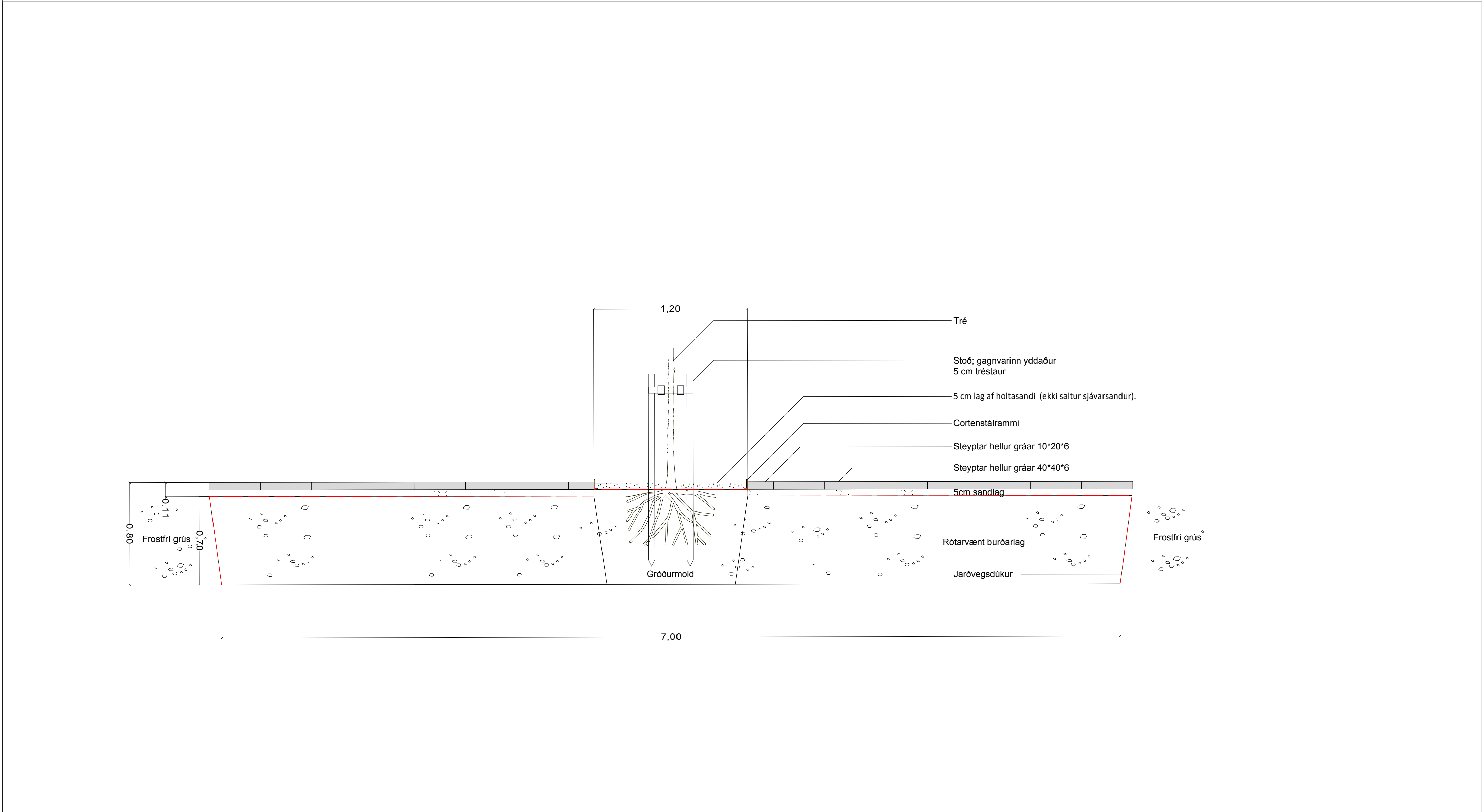
Deiliteikning 6; 1:20
