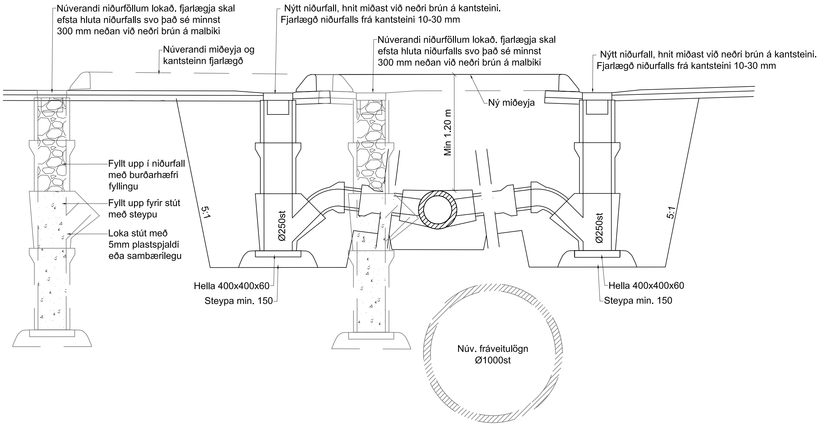
Frágangur niðurfalls, tvöfalt 1:20
