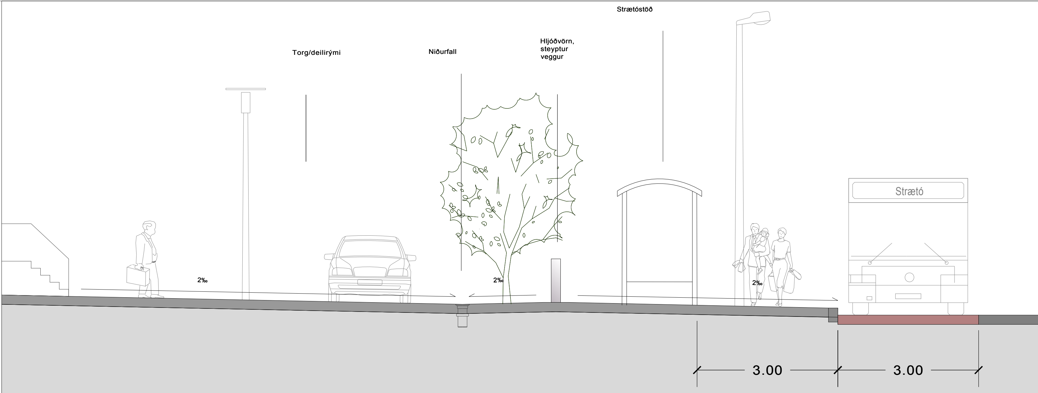
Kennisnið B-B; biðstöð við Reykjahlíð 1:50
