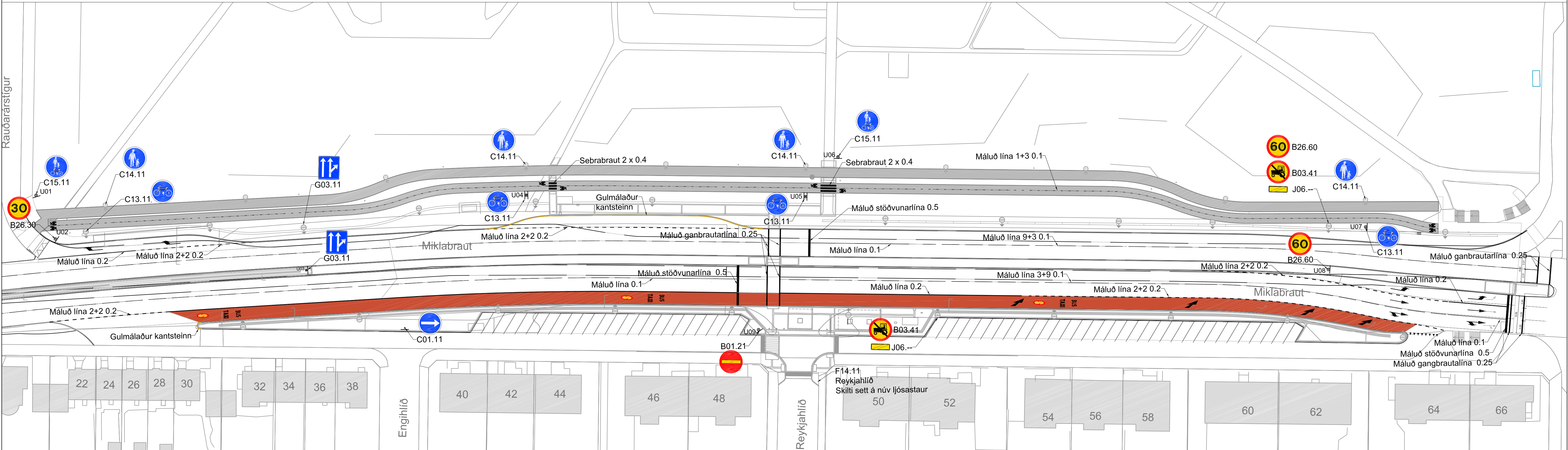
Grunnmynd 1:500
