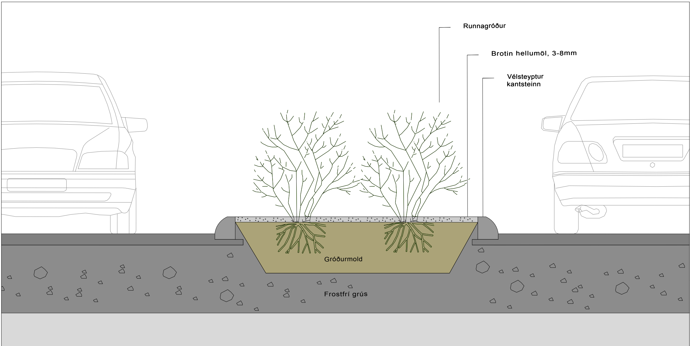
Miðeili kennisnið 1:20
