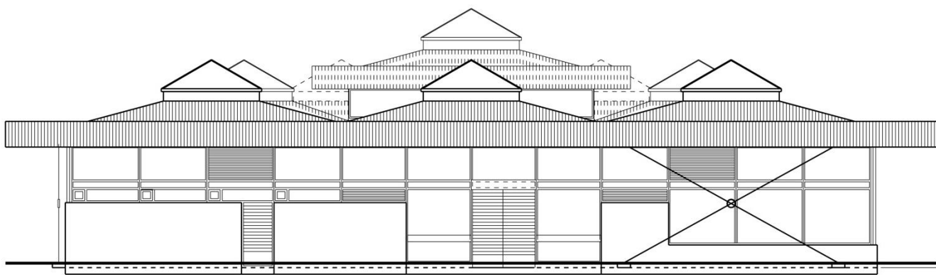
Útlit vesturhlið
