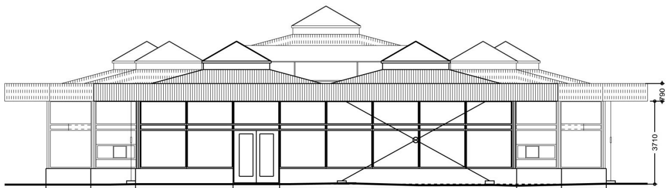
Útlit austurhlið
